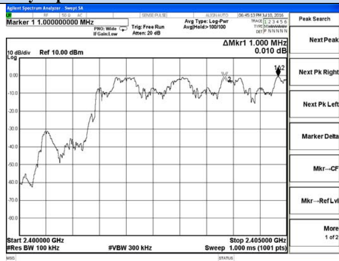
\pi/4 DQPSK(2Mbps)
