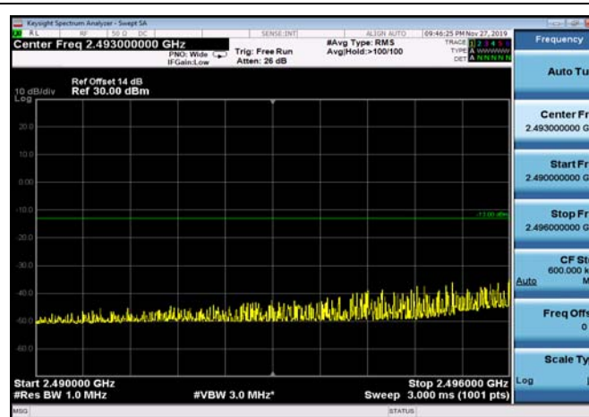
FDD07_5MHz_2502.5_Q16_OneRB_low _ExtraBands_Range_2490~2496
