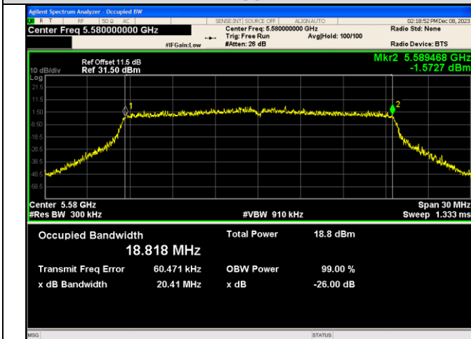
IEEE 802.11ax_Channel 116_20MHz_Antenna 1_RU&amp;Index SU
