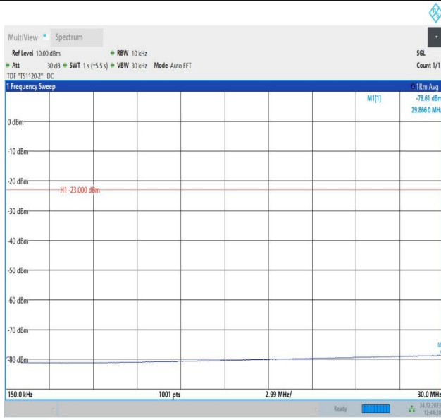
5-5-10MHz-10MHz-QPSK-QPSK-20501-20600-50RB#0-50RB #0-0.15~30MHz-PASS
