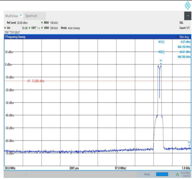
5-5-10MHz-10MHz-QPSK-QPSK-20476-20575-50RB#0-50RB #0-30~1000MHz-PASS
