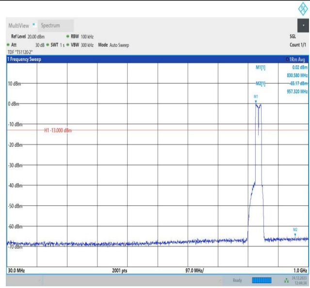
5-5-10MHz-10MHz-QPSK-QPSK-20501-20600-50RB#0-50RB #0-30~1000MHz-PASS
