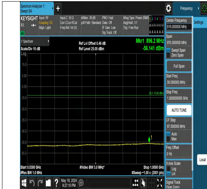
Band4-1413-3-30~1000MHz-PASS
