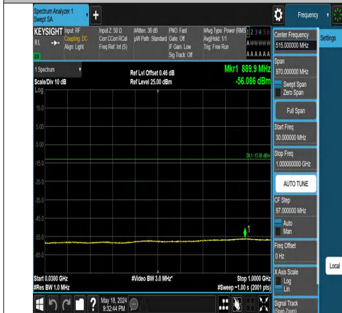
Band4-1513-5-30~1000MHz-PASS
