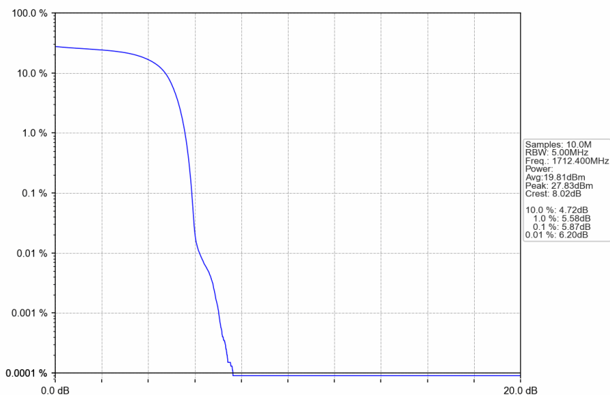
Band4_HSUPA_LCH_1712.4MHz_Subtest 1_NTNV
