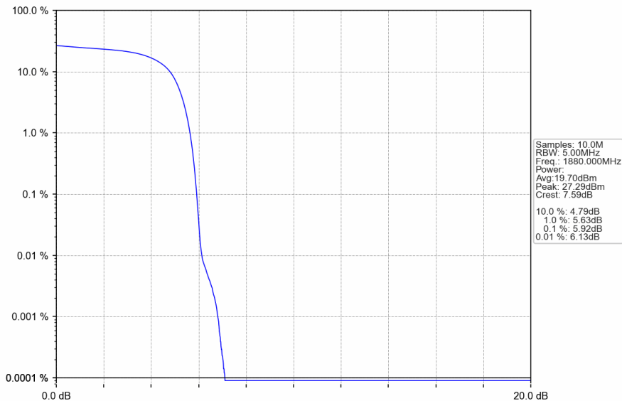
Band2_HSUPA_MCH_1880MHz_Subtest 1_NTNV
