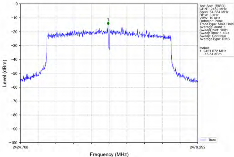
802.11ax(HE40)_HCH_2452MHz_RU484_Left_Ant1 (SISO)_NTNV
