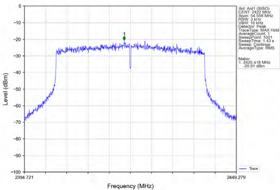
802.11ax(HE40)_LCH_2422MHz_RU484_Left_Ant1 (SISO)_NTNV
