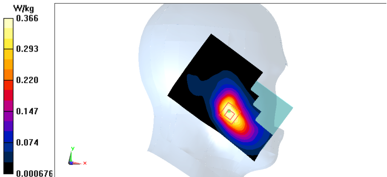
Fig.13 LTE Band7
