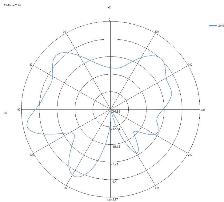
XZ-plane
