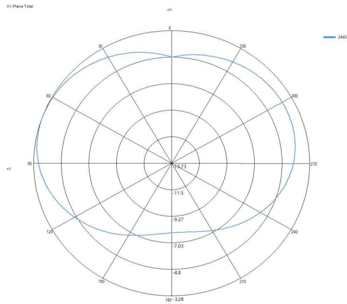
XY-plane
