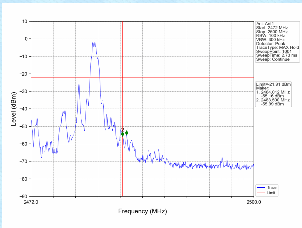
GFSK_HCH_2480MHz_Ant1_NTNV
