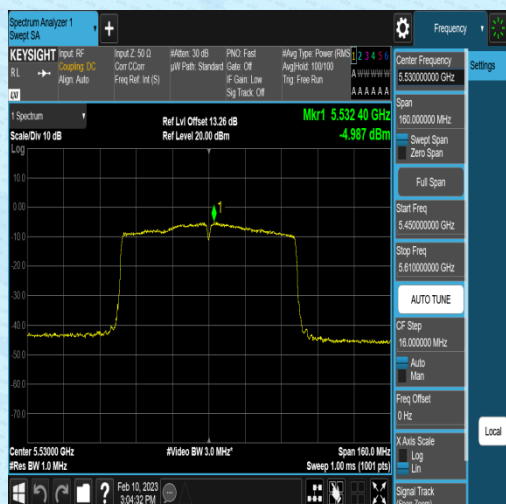
11AC80SISO-Ant2-5530--5.49-0.50-0.00-0.00
