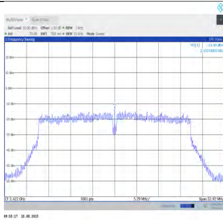
11n40MIMO-Ant10-2422
