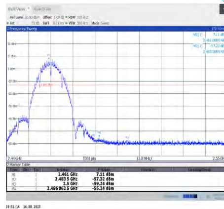
11b-CDD-Ant8-2462
