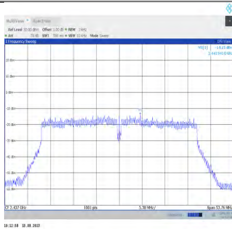
11n40MIMO-Ant10-2437
