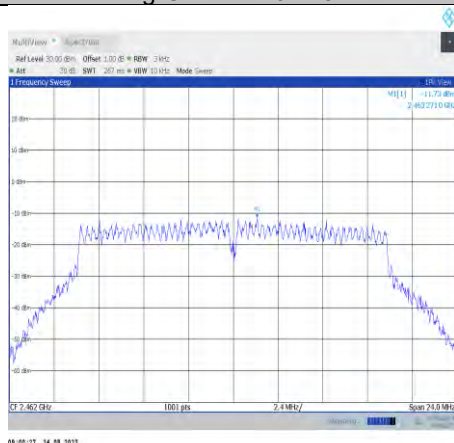
11g-CDD-Ant10-2462
