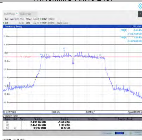
11n40MIMO-Ant10-2452
