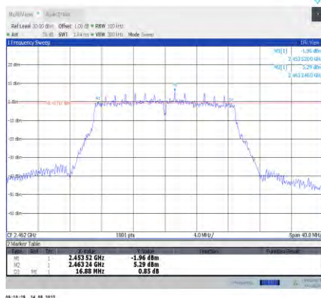
11n20MIMO-Ant10-2462
