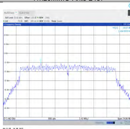
11n20MIMO-Ant8-2462
