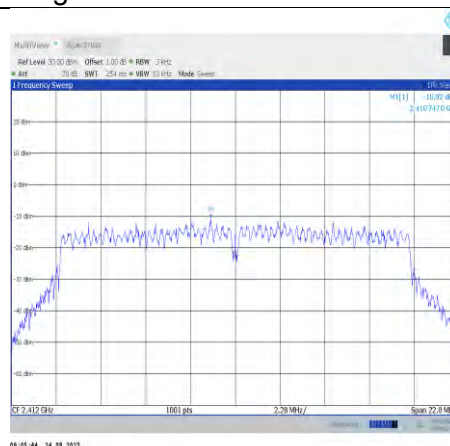
11n20MIMO-Ant8-2412
