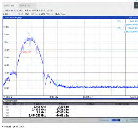
11b-CDD-Ant10-2462
