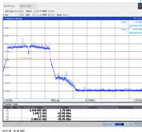
11n40MIMO-Ant10-2452
