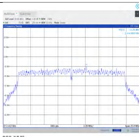
11n20MIMO-Ant10-2412
