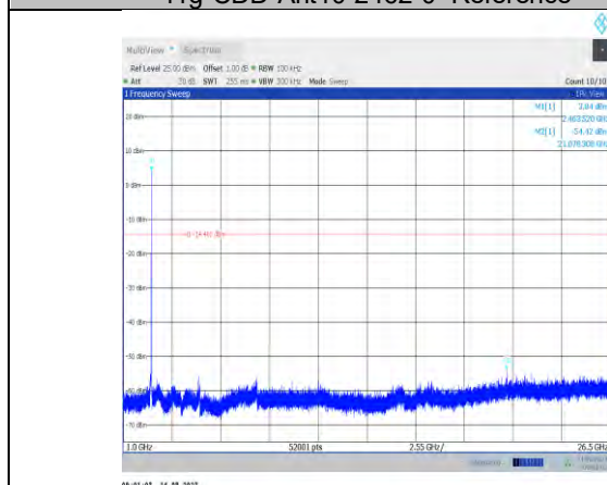
11g-CDD-Ant10-2462-1000~26500
