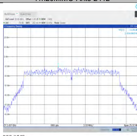
11n20MIMO-Ant8-2437
