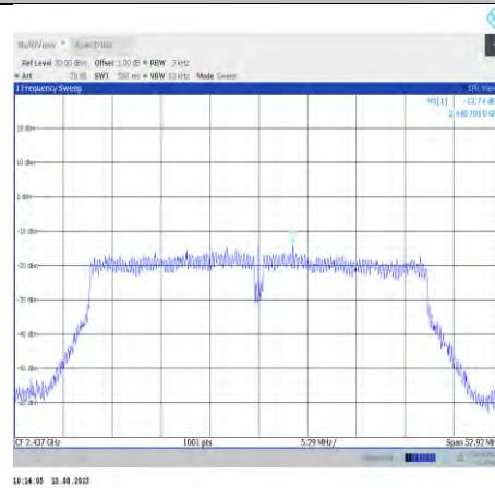
11n40MIMO-Ant8-2437
