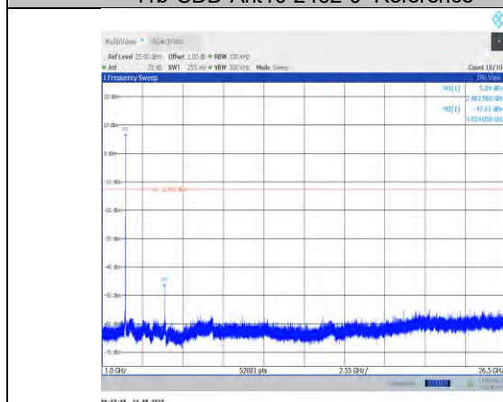
11b-CDD-Ant10-2462-1000~26500
