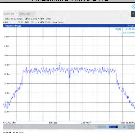
11n20MIMO-Ant10-2437
