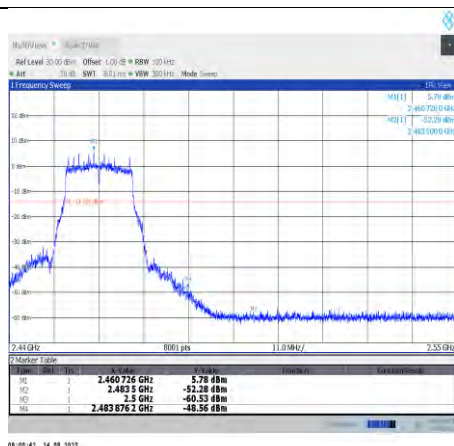
11g-CDD-Ant10-2462
