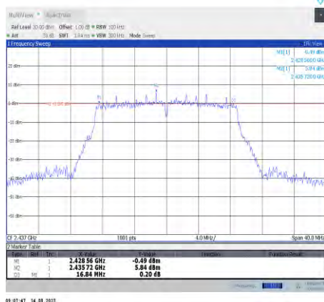
11n20MIMO-Ant10-2437
