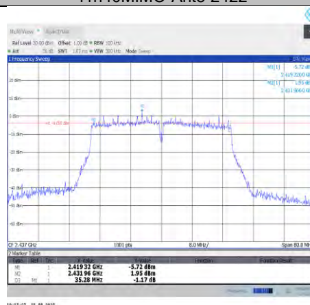
11n40MIMO-Ant8-2437
