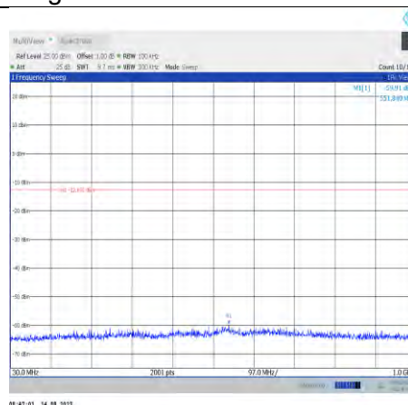
11b-CDD-Ant10-2462-30~1000
