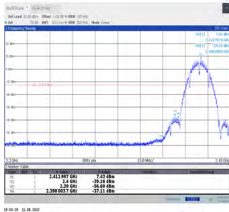
11b-CDD-Ant10-2412
