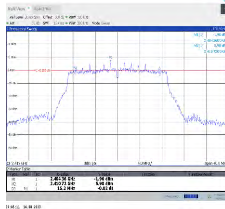
11n20MIMO-Ant8-2412
