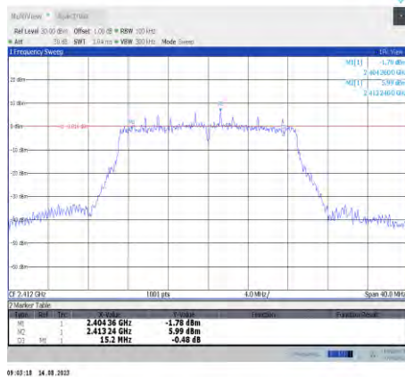
11n20MIMO-Ant10-2412
