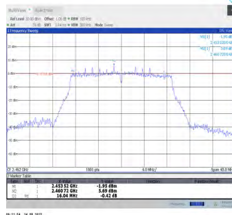
11n20MIMO-Ant8-2462
