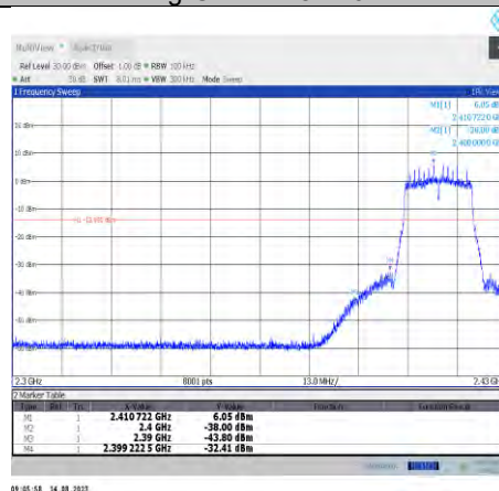
11n20MIMO-Ant8-2412
