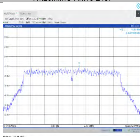
11n20MIMO-Ant10-2462
