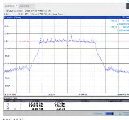
11n20MIMO-Ant8-2437
