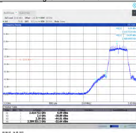
11n20MIMO-Ant10-2412
