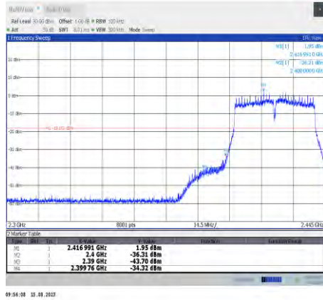
11n40MIMO-Ant10-2422
