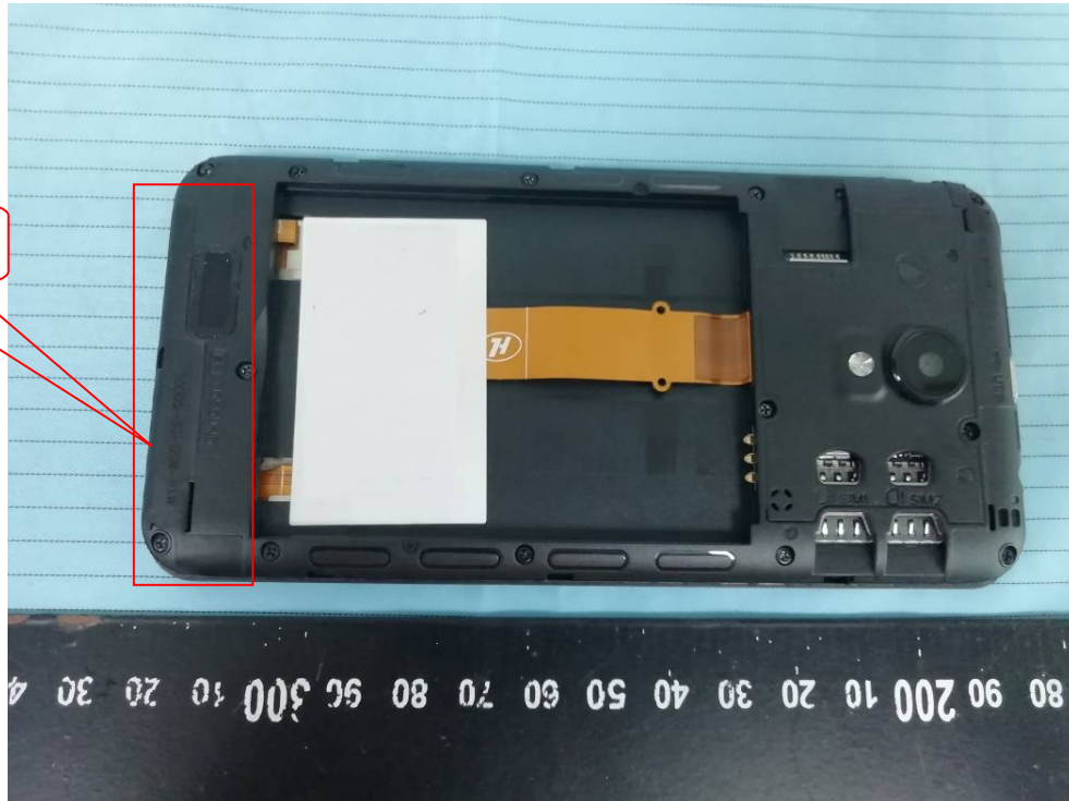
GSM&WCDMA Antenna
