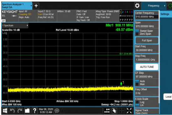
11G-Ant1-2412-30~1000-PASS
