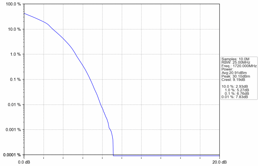
Band4_20MHz_16QAM_LCH_1720MHz_RB_27_0_NTNV
