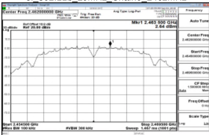
Reference Level el 802.11b 20MHz Chain0 2462MHz
