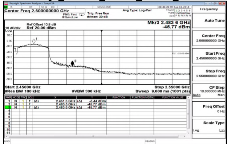
Band Edge 802.11n 40MHz Chain0 2452MHz
