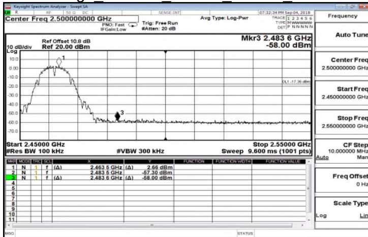
Band Edge 802.11b 20MHz Chain0 2462MHz
