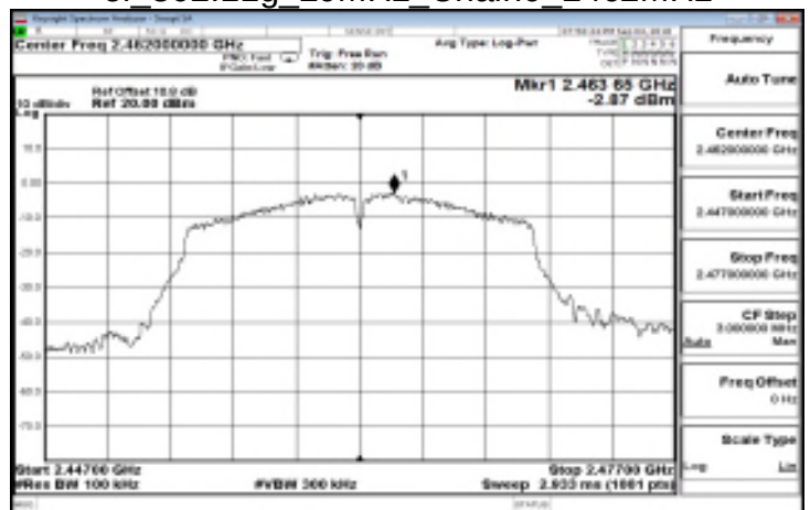
Reference Level el 802.11g 20MHz Chain0 2462MHz
