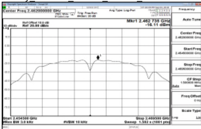
Power Density 802.11b 20MHz Chain0 2462MHz
