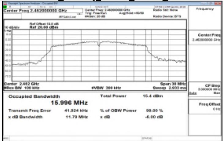
OBW 6dB_802.11g_20MHz_Chain0_2462MHz
