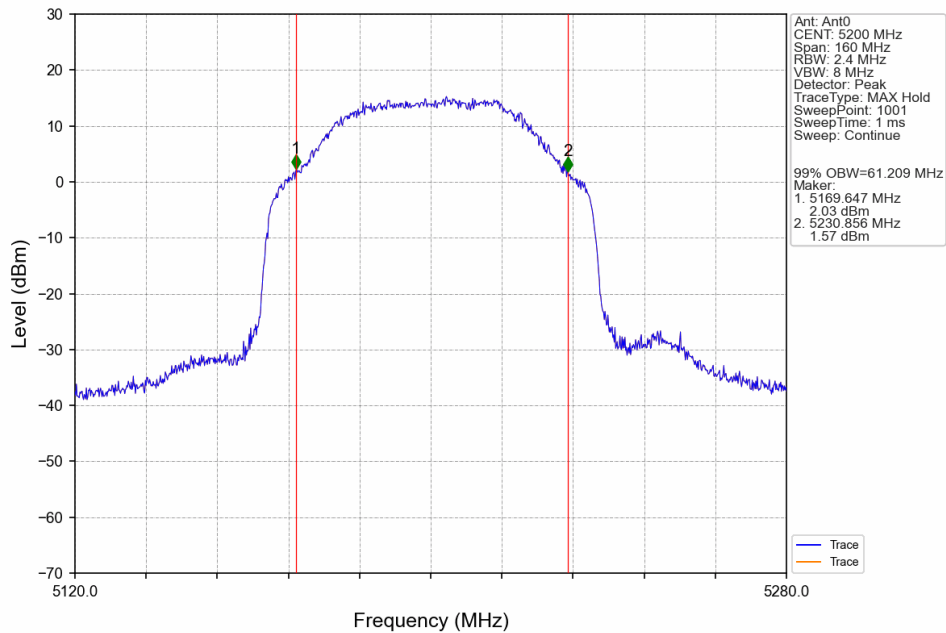
80M_MCH_5200MHz_Ant0_NTNV
