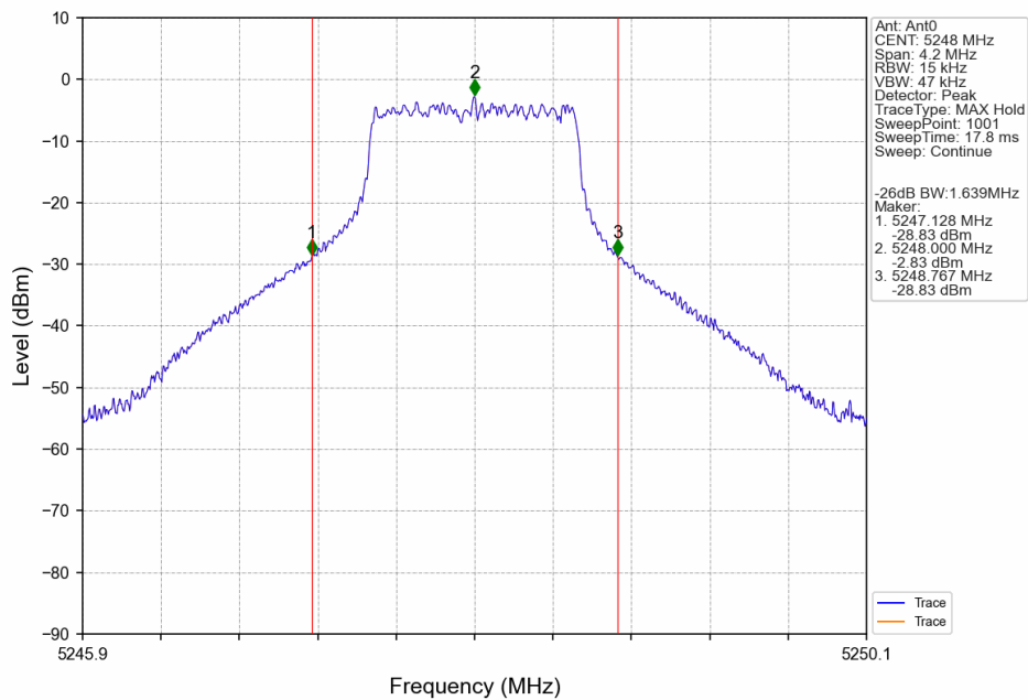
1.4M_HCH_5248MHz_Ant0_NTNV
