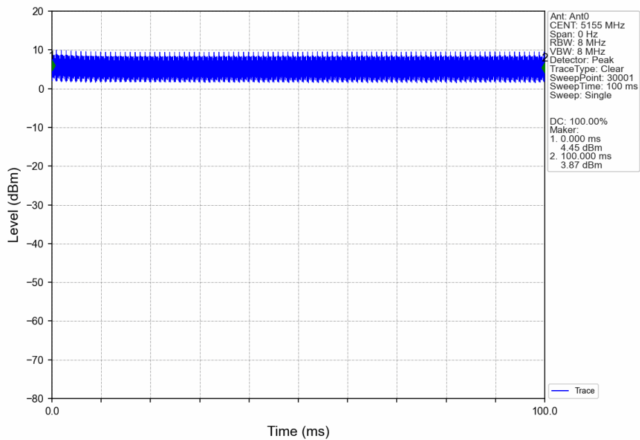
5M_LCH_5155MHz_Ant0_NTNV
