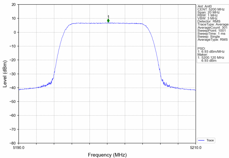
10M_MCH_5200MHz_Ant0_NTNV
