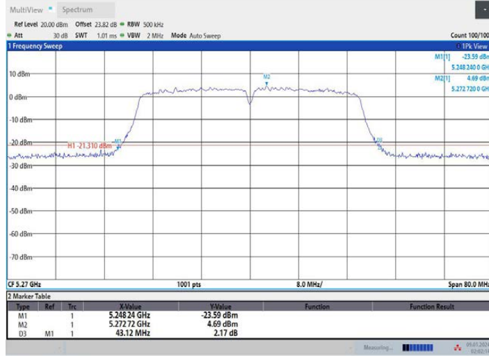
11AC40MIMO_Ant2_5270
