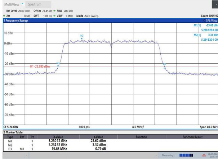
11N20MIMO_Ant2_5240
