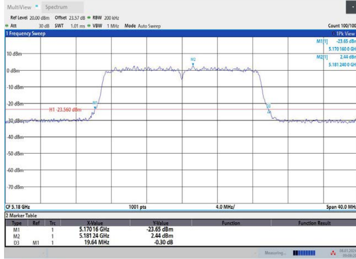
11N20MIMO_Ant2_5180
