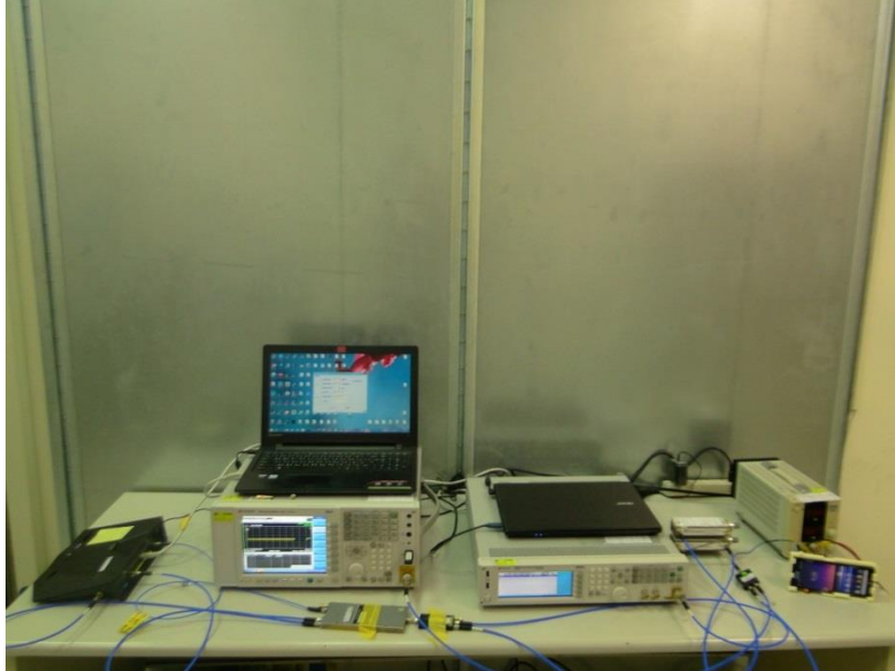
EUT
