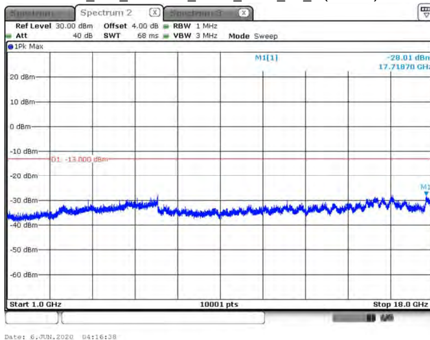
B26_15K_CH26788_BPSK_1RB0_TX_2 (Part 90)
