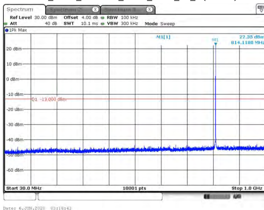
B26_3.75K_CH26692_BPSK_1RB0_TX_2 (Part 90)
