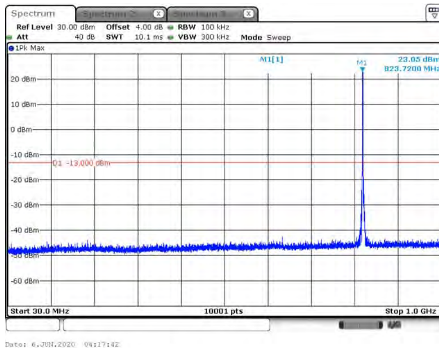
B26_15K_CH26788_BPSK_1RB0_TX_2 (Part 90)
