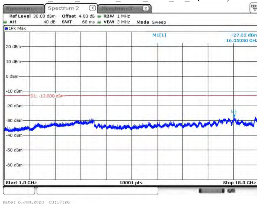
B26_3.75K_CH26692_BPSK_1RB0_TX_2 (Part 90)
