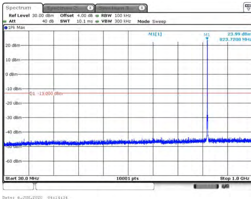
B26_15K_CH26788_QPSK_1RB0_TX_2 (Part 90)
