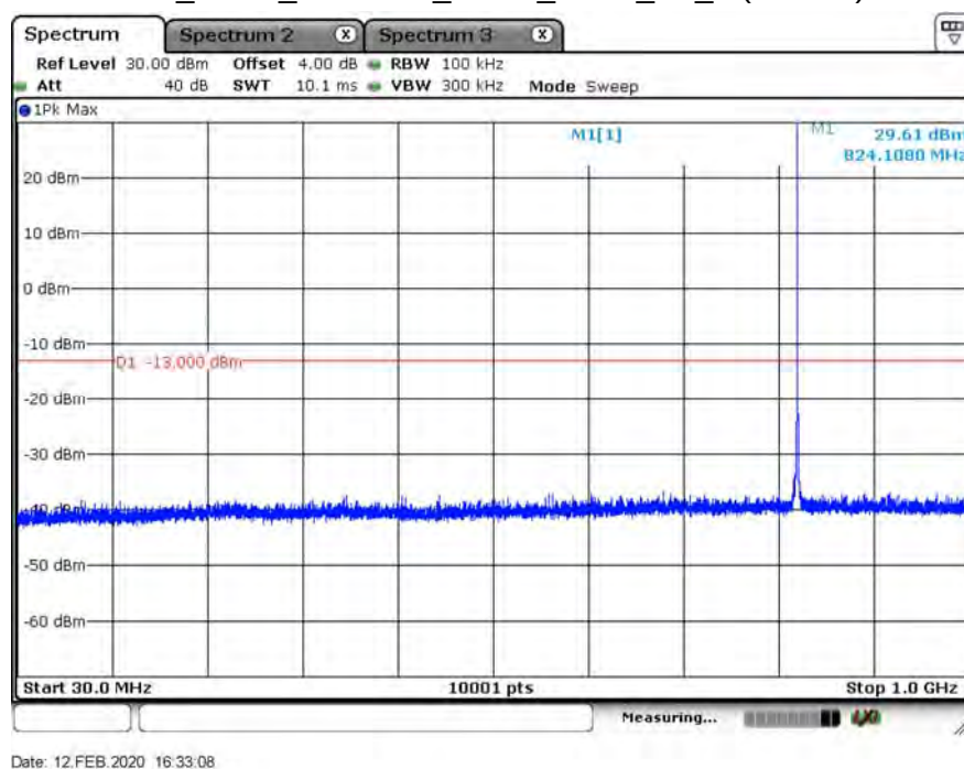
B26_3.75K_CH26792_BPSK_1RB0_TX_2 (Part 22)
