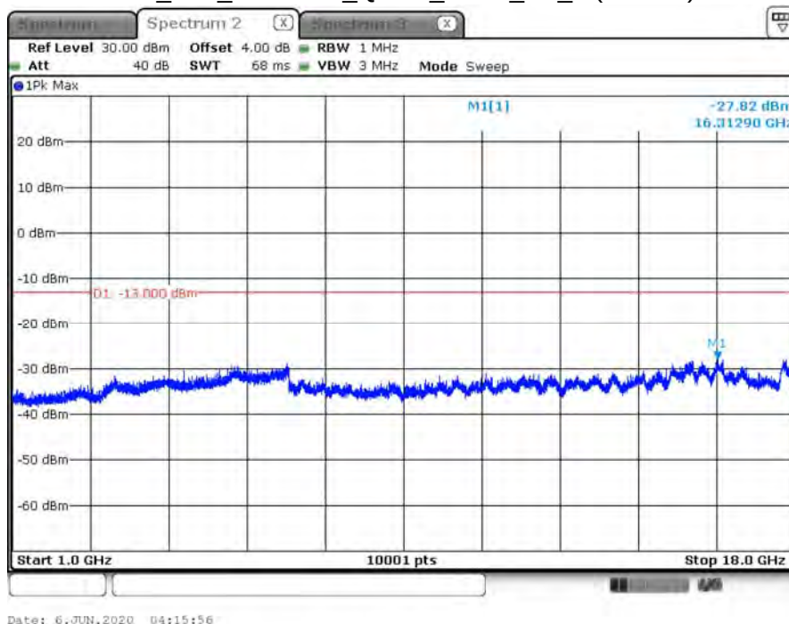
B26_15K_CH26788_QPSK_1RB0_TX_2 (Part 90)
