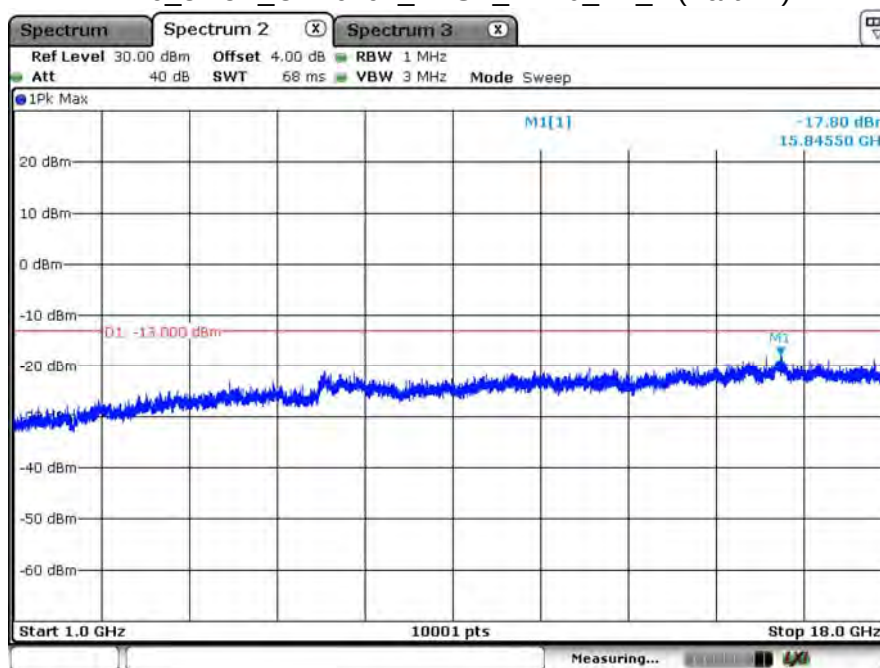
B26_3.75K_CH26792_BPSK_1RB0_TX_2 (Part 22)
