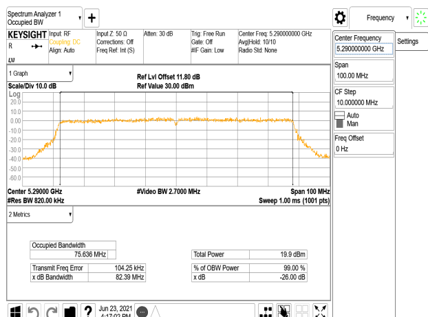
802.11ac_80MHz_Chain1_5290MHz
