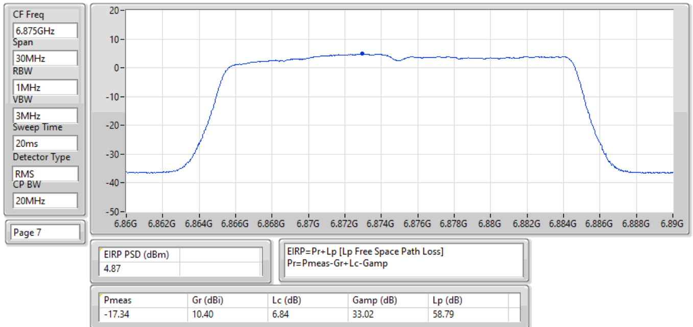
EIRP PSD;Band:6.7G;be20,BF;BWch:20MHz;Nss:1,(M0);Nant:4;Ch:6875MHz;TX
