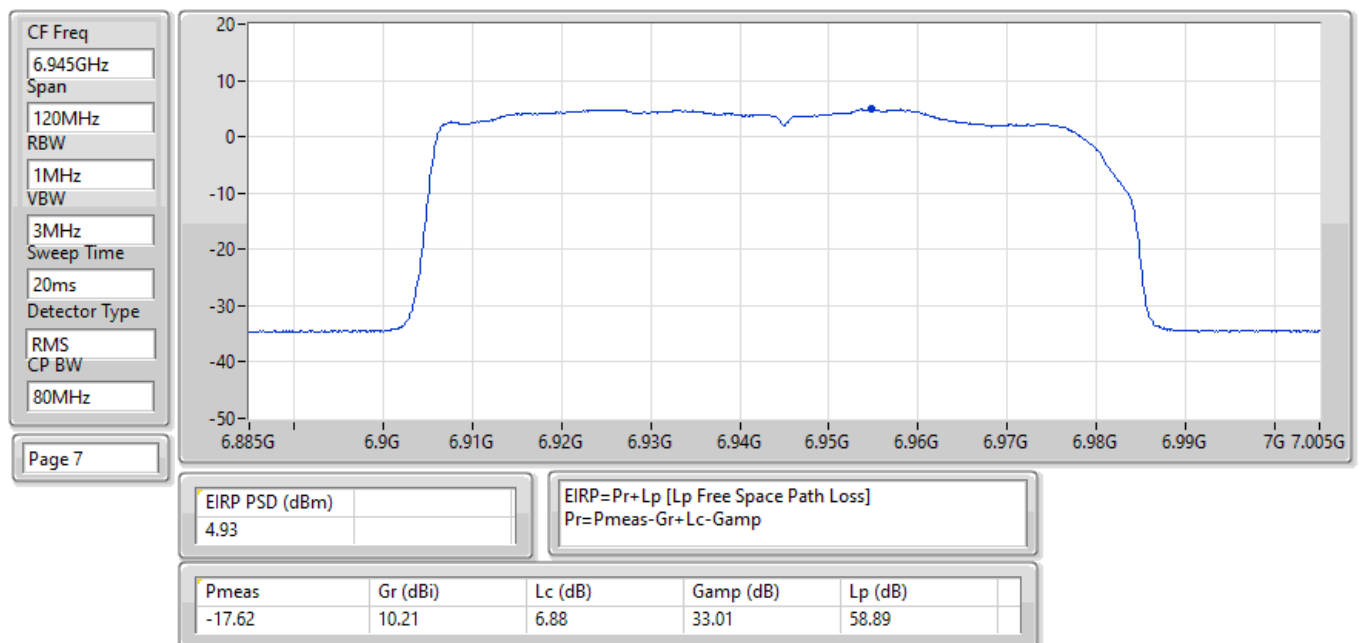
EIRP PSD;Band:7.0G;be80,BF;BWch:80MHz;Nss:1,(M0);Nant:4;Ch:6945MHz;TX
