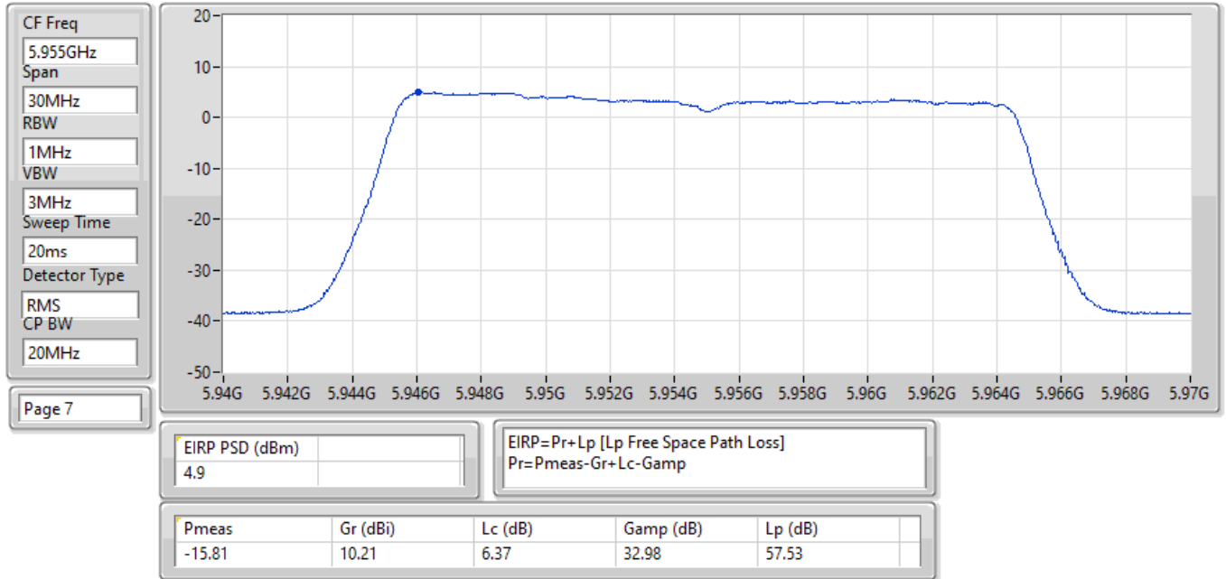
EIRP PSD;Band:6.2G;be20,BF;BWch:20MHz;Nss:1,(M0);Nant:4;Ch:5955MHz;TX
