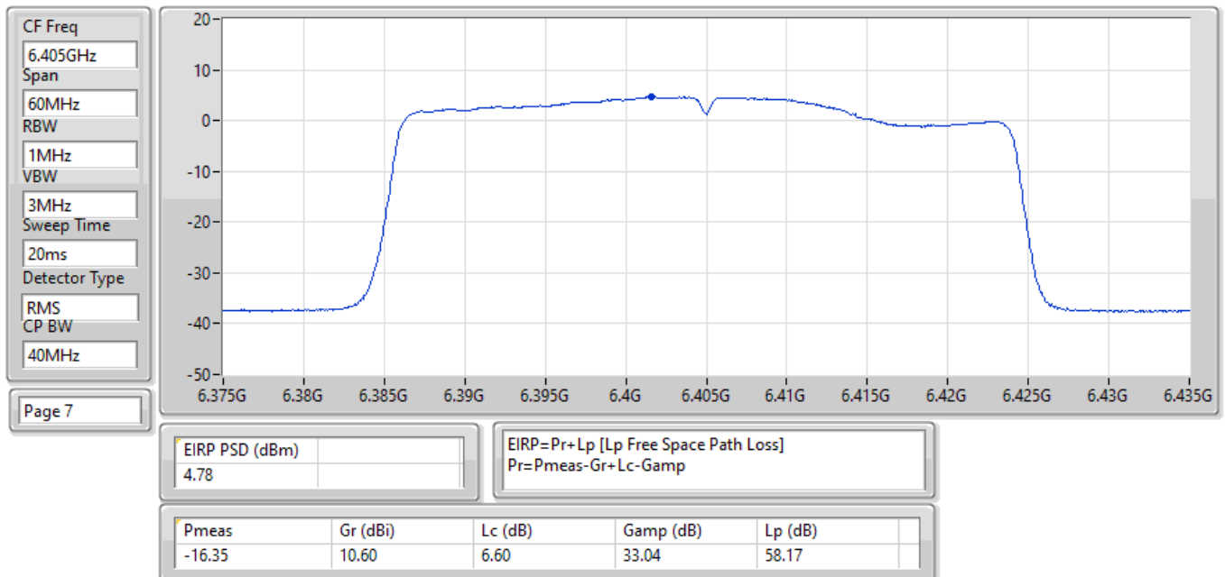
EIRP PSD;Band:6.2G;be40,BF;BWch:40MHz;Nss:1,(M0);Nant:4;Ch:6405MHz;TX
