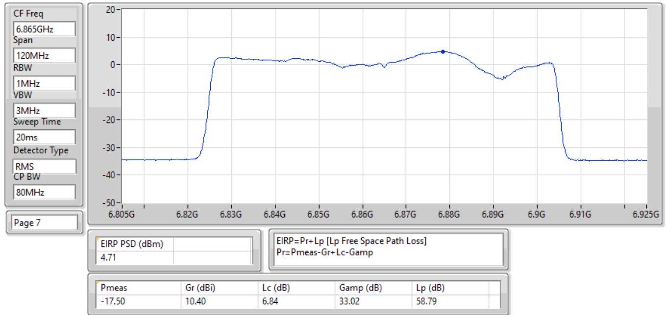
EIRP PSD;Band:6.7G;be80,BF;BWch:80MHz;Nss:1,(M0);Nant:4;Ch:6865MHz;TX
