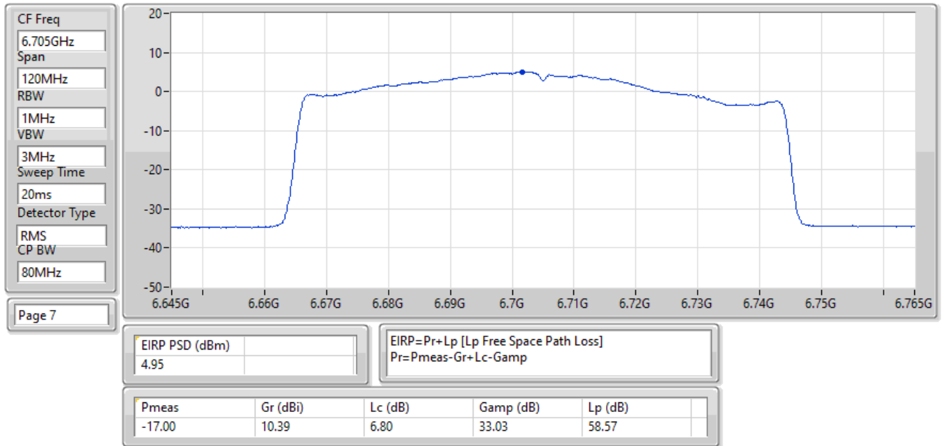
EIRP PSD;Band:6.7G;be80,BF;BWch:80MHz;Nss:1,(M0);Nant:4;Ch:6705MHz;TX
