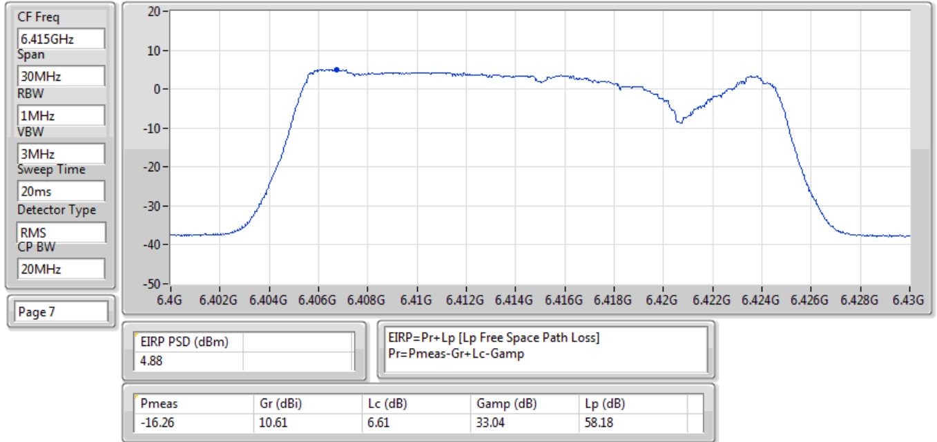
EIRP PSD;Band:6.2G;be20,BF;BWch:20MHz;Nss:1,(M0);Nant:4;Ch:6415MHz;TX
