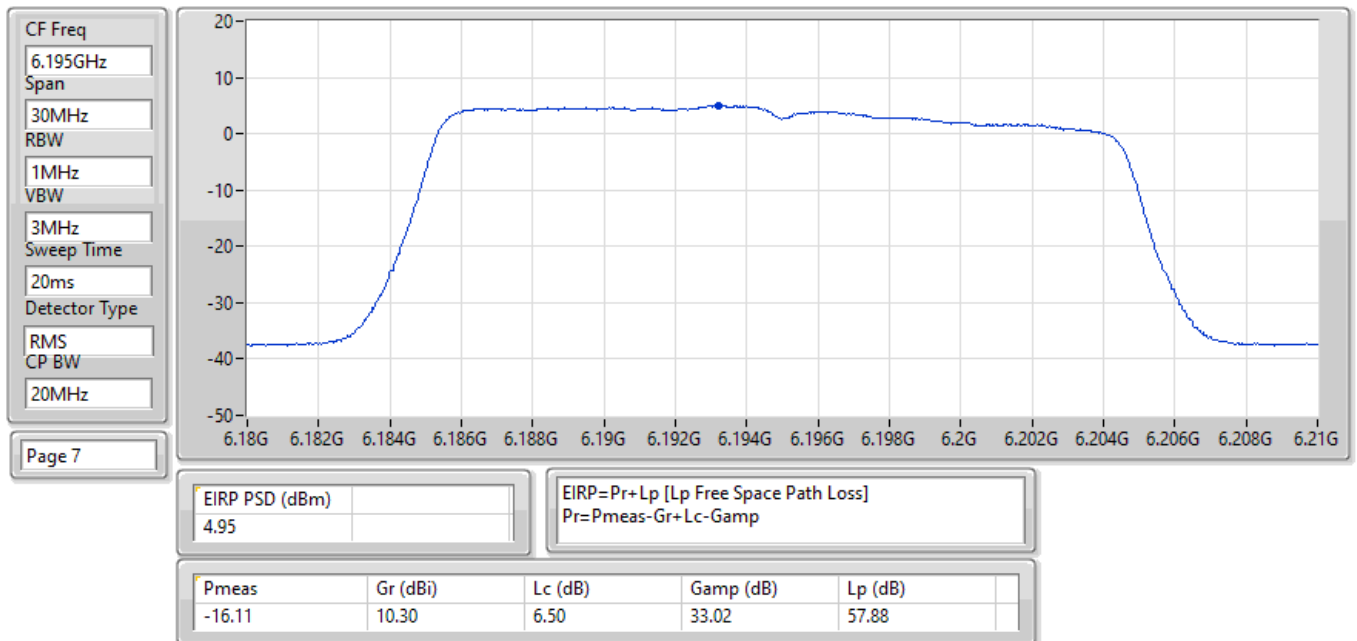
EIRP PSD;Band:6.2G;be20,BF;BWch:20MHz;Nss:1,(M0);Nant:4;Ch:6195MHz;TX
