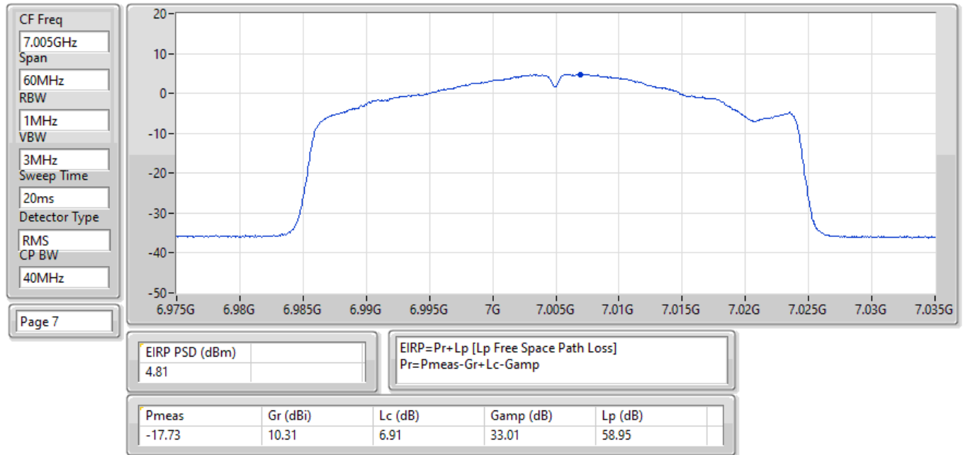
EIRP PSD;Band:7.0G;be40,BF;BWch:40MHz;Nss:1,(M0);Nant:4;Ch:7005MHz;TX
