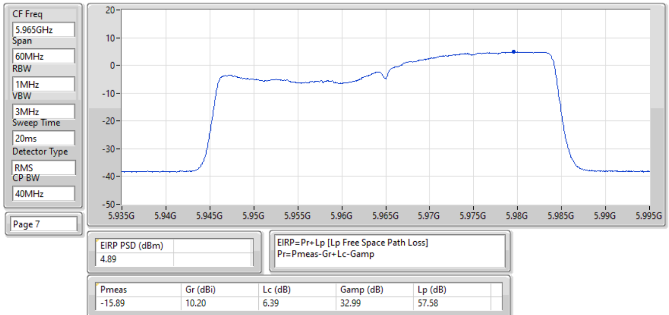
EIRP PSD;Band:6.2G;be40,BF;BWch:40MHz;Nss:1,(M0);Nant:4;Ch:5965MHz;TX
