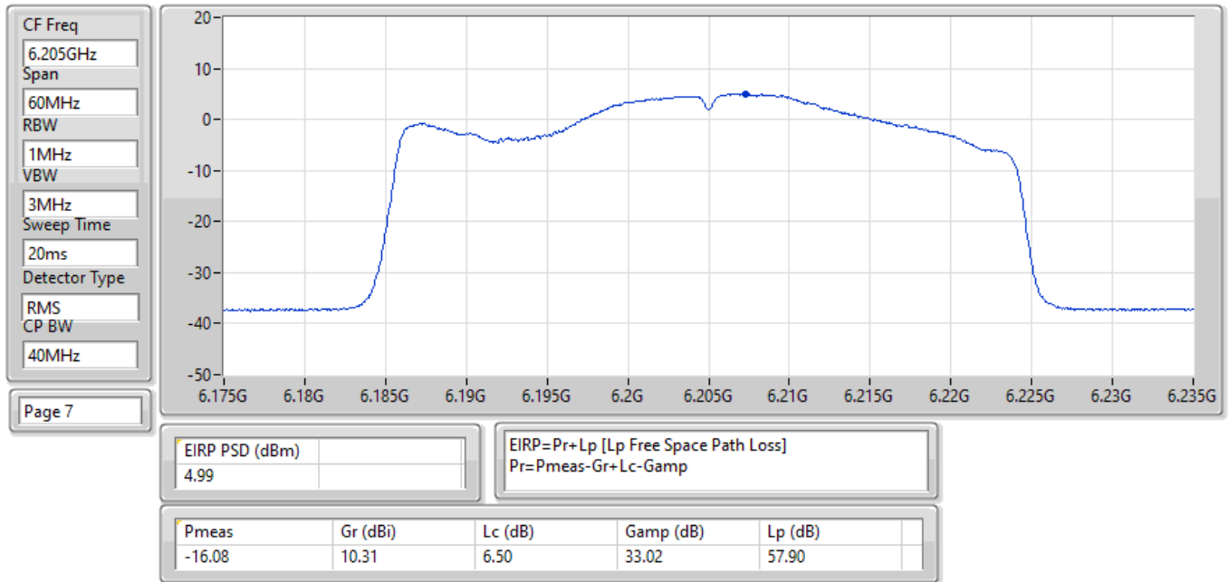
EIRP PSD;Band:6.2G;be40,BF;BWch:40MHz;Nss:1,(M0);Nant:4;Ch:6205MHz;TX
