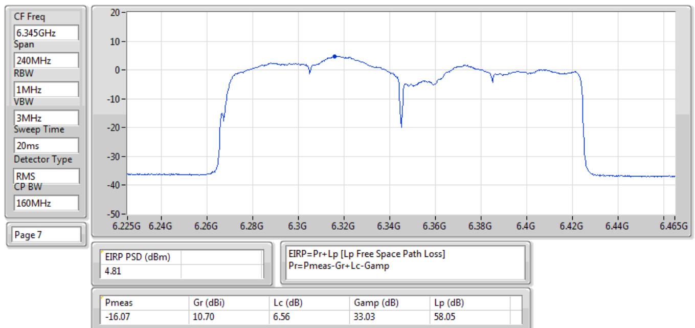
EIRP PSD;Band:6.2G;be160,BF;BWch:160MHz;Nss:1,(M0);Nant:4;Ch:6345MHz;TX
