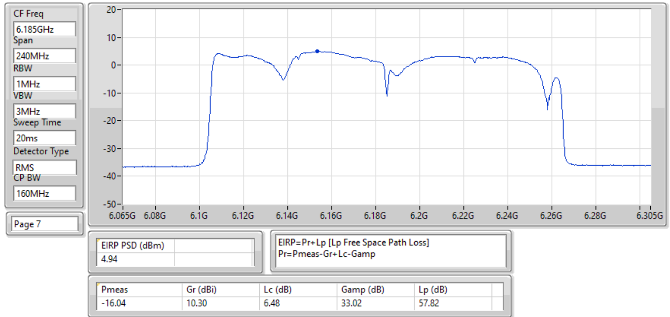
EIRP PSD;Band:6.2G;be160,BF;BWch:160MHz;Nss:1,(M0);Nant:4;Ch:6185MHz;TX
