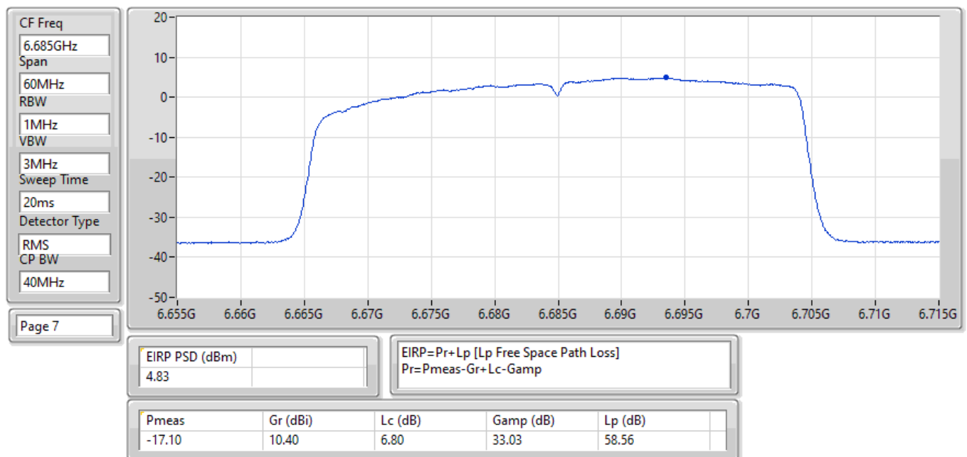
EIRP PSD;Band:6.7G;be40,BF;BWch:40MHz;Nss:1,(M0);Nant:4;Ch:6685MHz;TX
