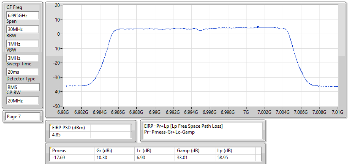
EIRP PSD;Band:7.0G;be20,BF;BWch:20MHz;Nss:1,(M0);Nant:4;Ch:6995MHz;TX
