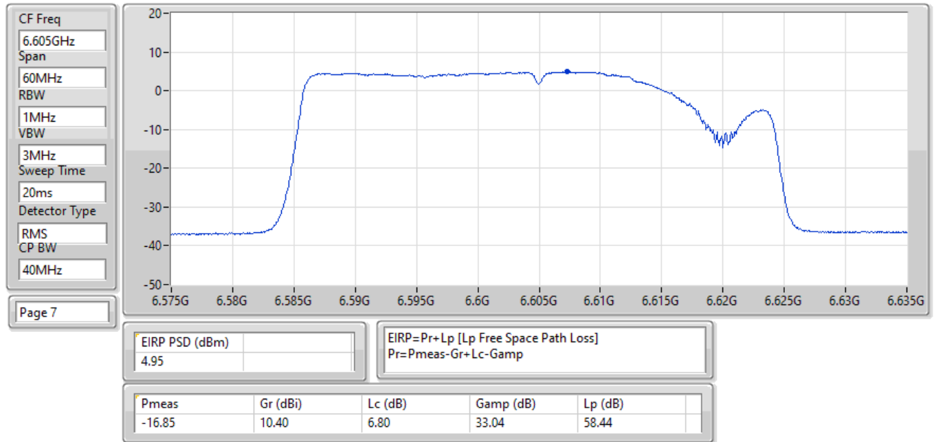
EIRP PSD;Band:6.7G;be40,BF;BWch:40MHz;Nss:1,(M0);Nant:4;Ch:6605MHz;TX
