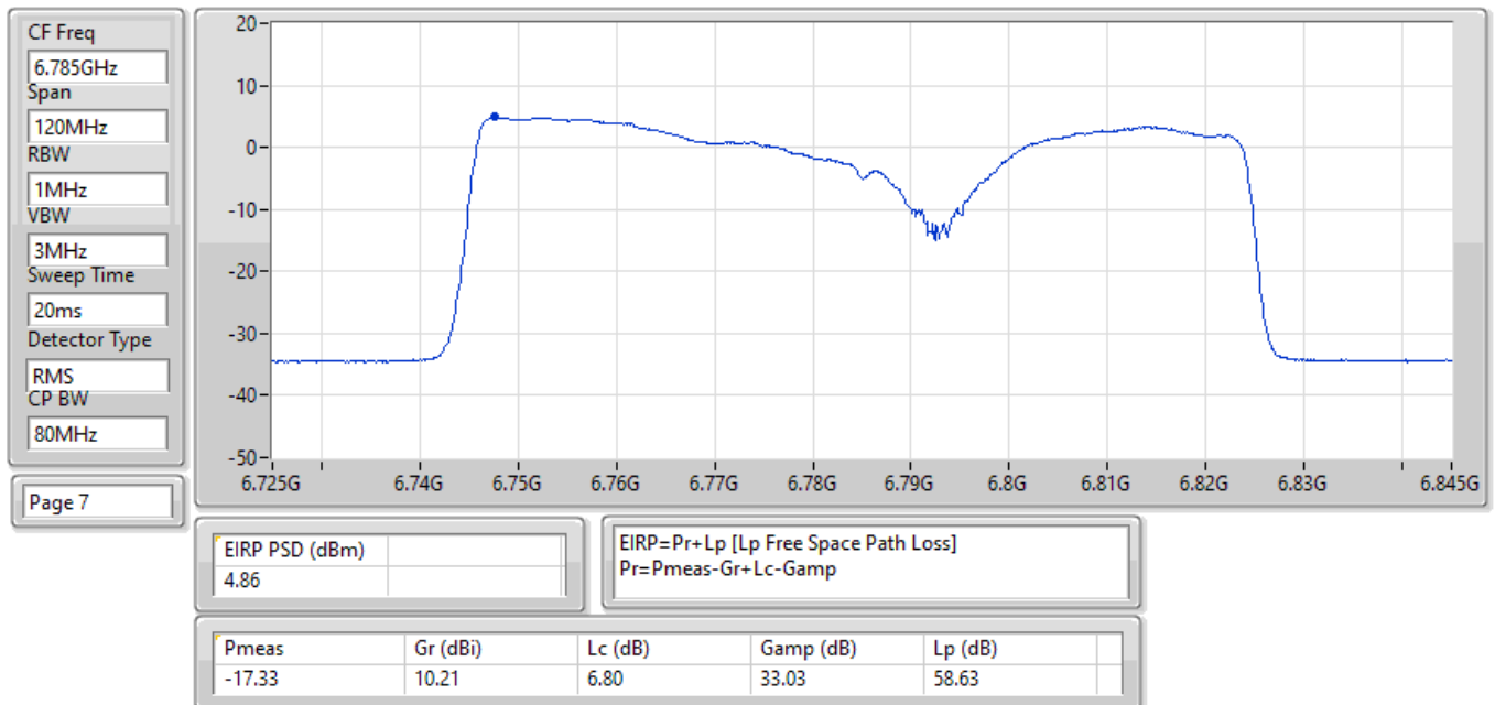
EIRP PSD;Band:6.7G;be80,BF;BWch:80MHz;Nss:1,(M0);Nant:4;Ch:6785MHz;TX
