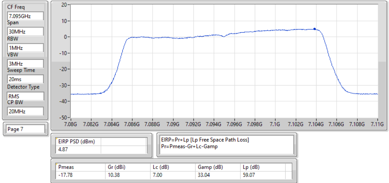
EIRP PSD;Band:7.0G;be20,BF;BWch:20MHz;Nss:1,(M0);Nant:4;Ch:7095MHz;TX
