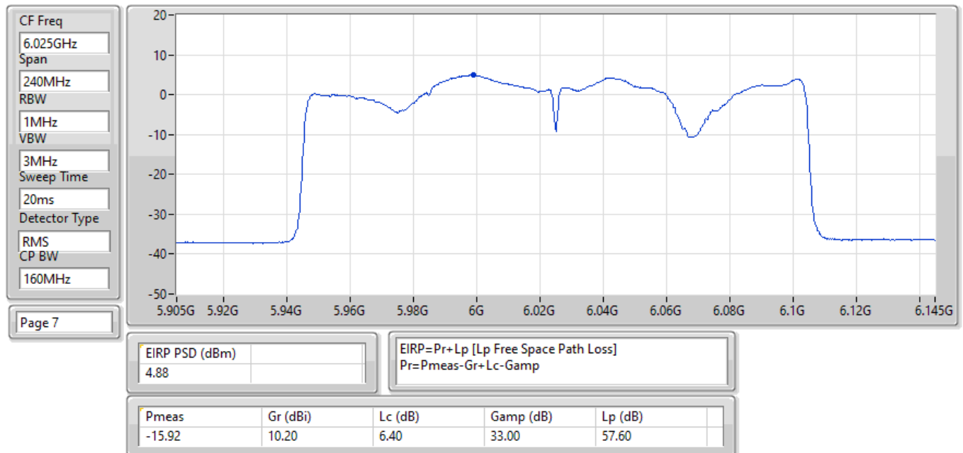
EIRP PSD;Band:6.2G;be160,BF;BWch:160MHz;Nss:1,(M0);Nant:4;Ch:6025MHz;TX
