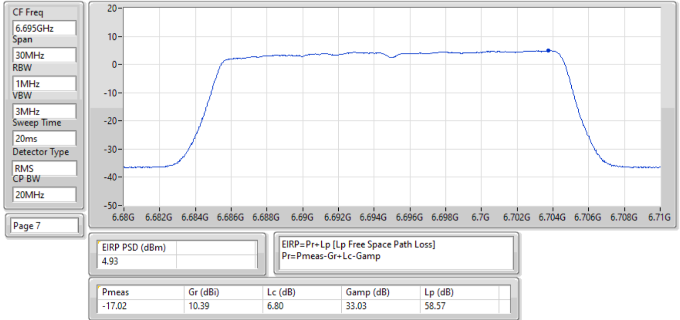
EIRP PSD;Band:6.7G;be20,BF;BWch:20MHz;Nss:1,(M0);Nant:4;Ch:6695MHz;TX
