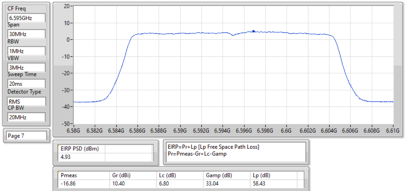
EIRP PSD;Band:6.7G;be20,BF;BWch:20MHz;Nss:1,(M0);Nant:4;Ch:6595MHz;TX
