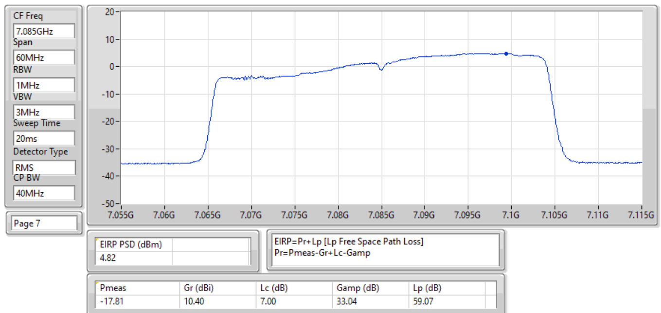
EIRP PSD;Band:7.0G;be40,BF;BWch:40MHz;Nss:1,(M0);Nant:4;Ch:7085MHz;TX
