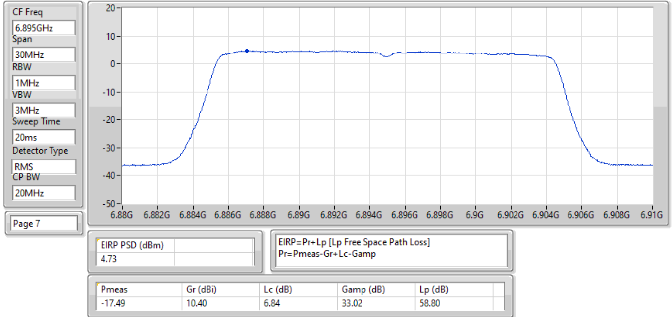
EIRP PSD;Band:7.0G;be20,BF;BWch:20MHz;Nss:1,(M0);Nant:4;Ch:6895MHz;TX
