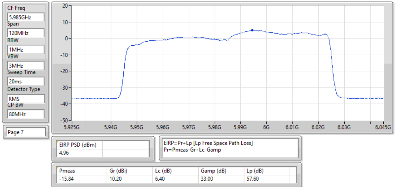
EIRP PSD;Band:6.2G;be80,BF;BWch:80MHz;Nss:1,(M0);Nant:4;Ch:5985MHz;TX
