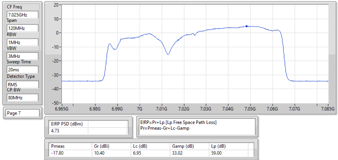
EIRP PSD;Band:7.0G;be80,BF;BWch:80MHz;Nss:1,(M0);Nant:4;Ch:7025MHz;TX
