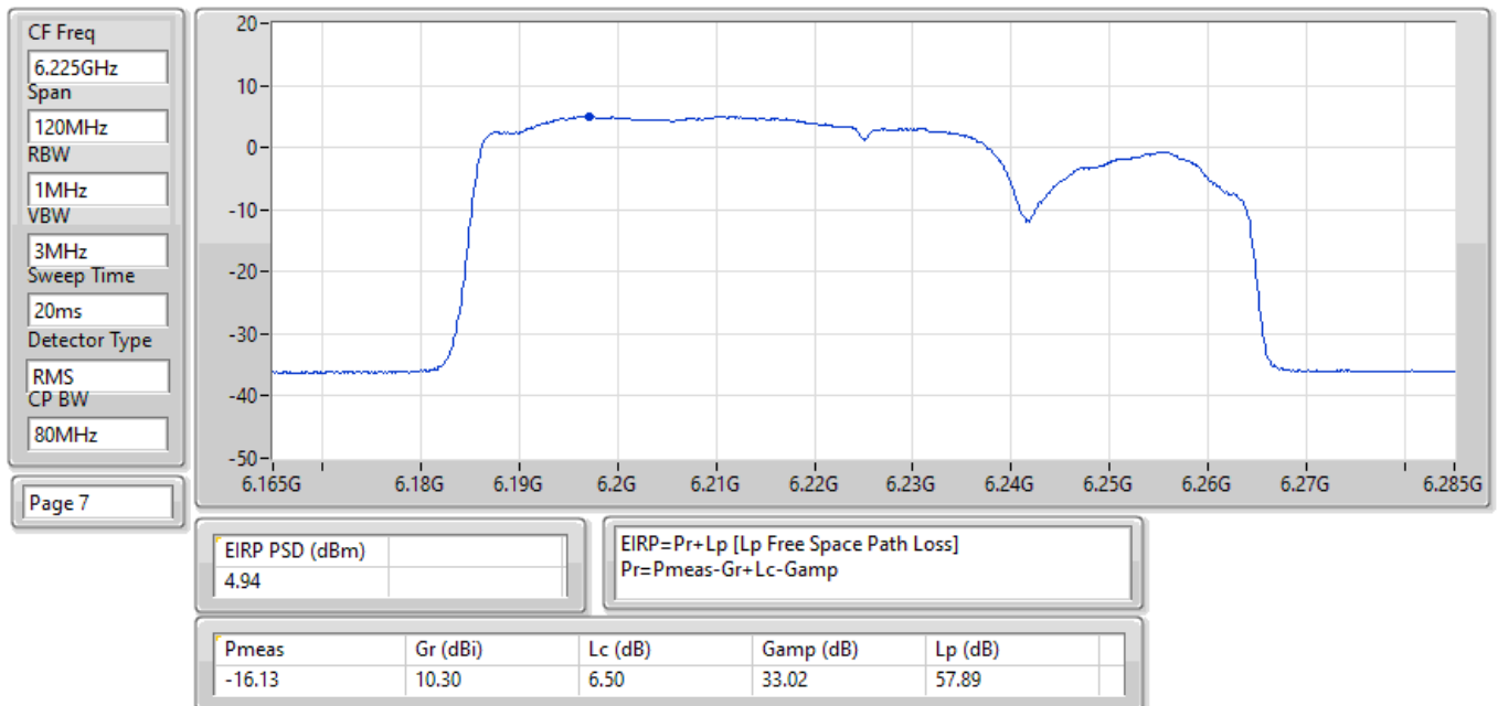
EIRP PSD;Band:6.2G;be80,BF;BWch:80MHz;Nss:1,(M0);Nant:4;Ch:6225MHz;TX
