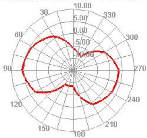
Bluetooth 78 TRP Phi=45
