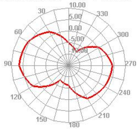
Bluetooth 37 TRP Phi=45
