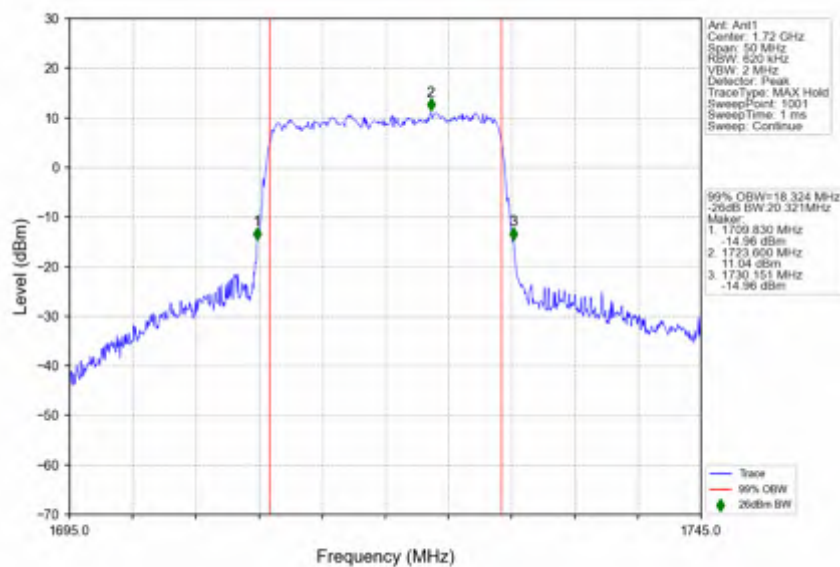
n66 30kHz SISO NTN 20MHz CP-OFDM 64 QAM 1720MHz Outer Full
