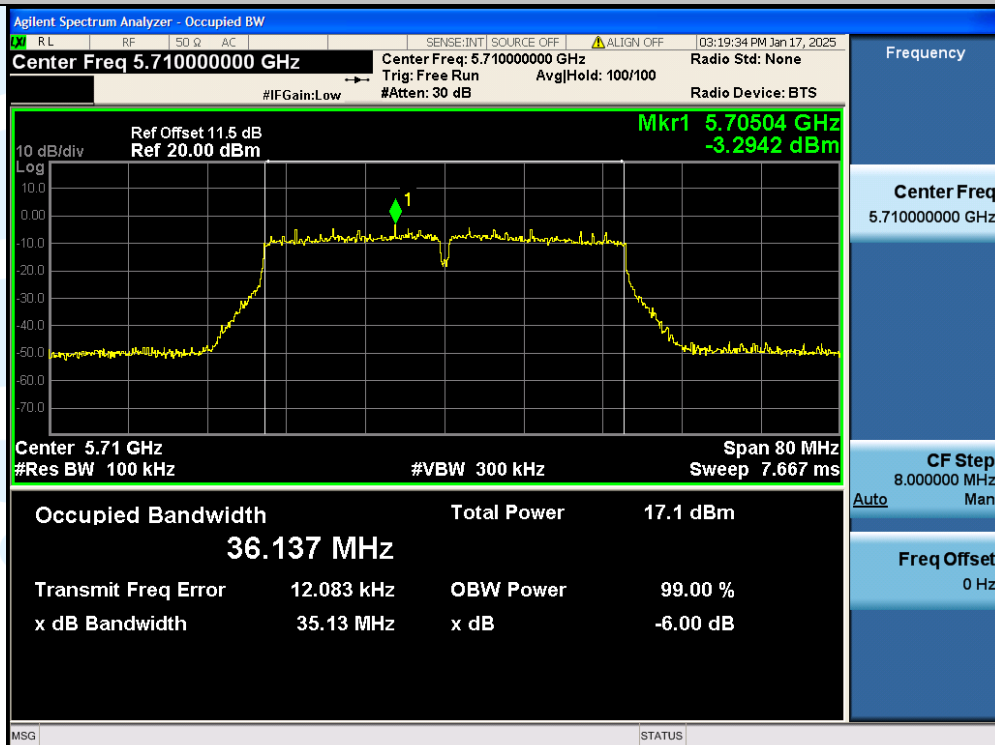
11N40SISO-Ant1-5710
