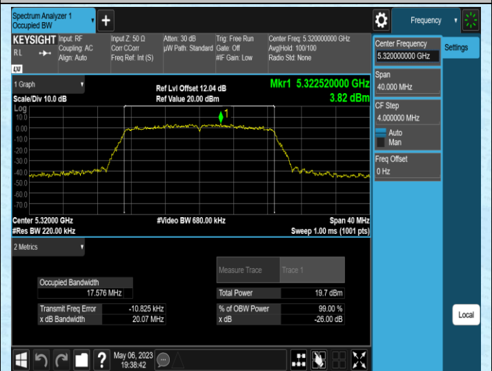
11N20MIMO-Ant1-5320
