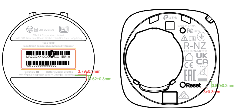
尺寸图
