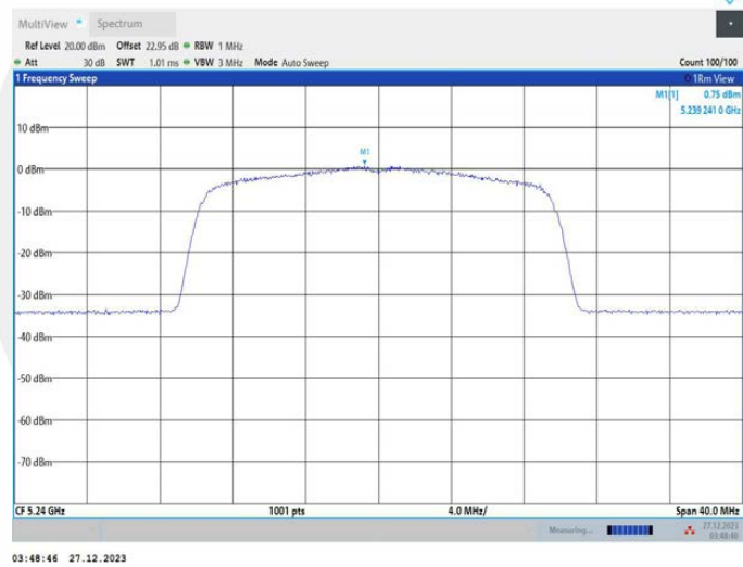
11AX20MIMO_Ant2_5240
