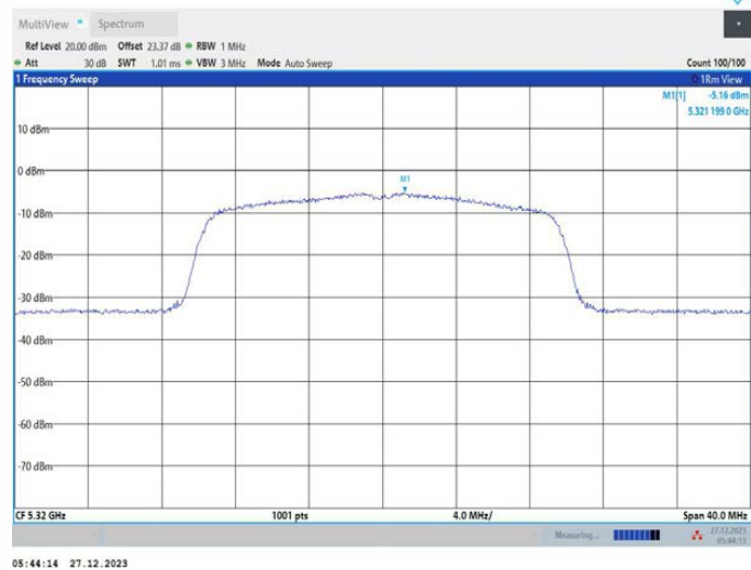
11AX20MIMO_Ant2_5320
