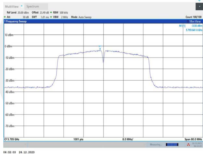
11N40MIMO_Ant4_5795
