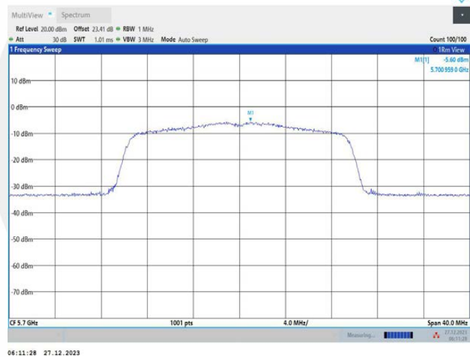
11AX20MIMO_Ant2_5700
