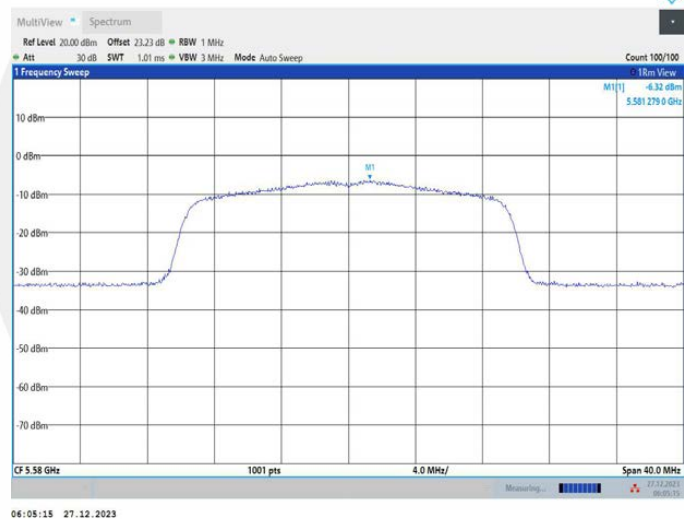
11AX20MIMO_Ant3_5580
