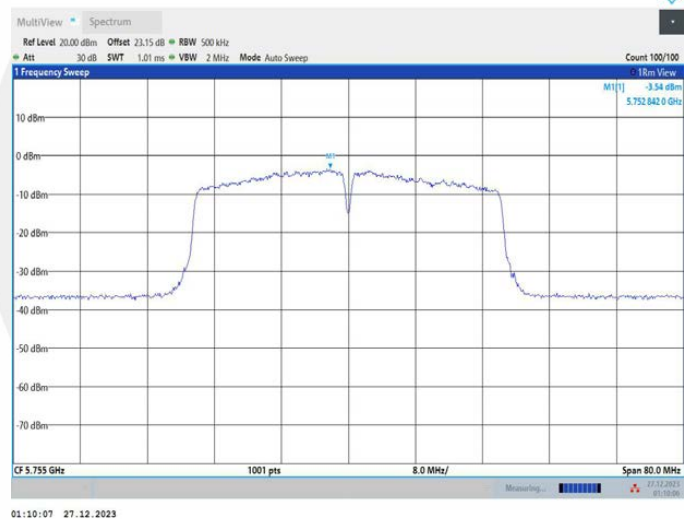
11AC40MIMO_Ant2_5755
