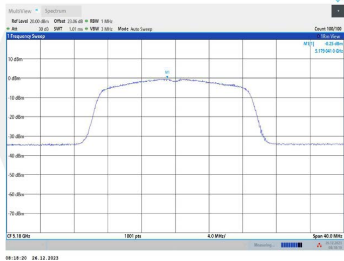
11AC20MIMO_Ant3_5180
