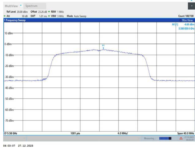
11AX20MIMO_Ant2_5580
