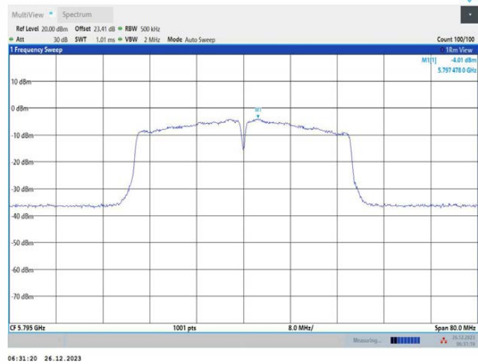
11N40MIMO_Ant3_5795
