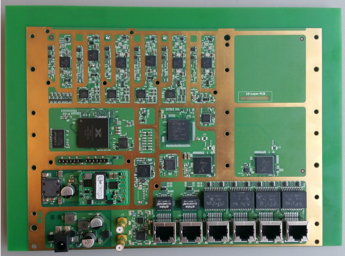
PCB Side_1_no shield – NU
