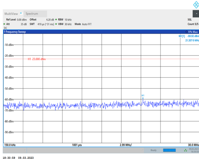
Band2-20MHz-QPSK-18700-1RB#0-Range2:0.15~30MHz
