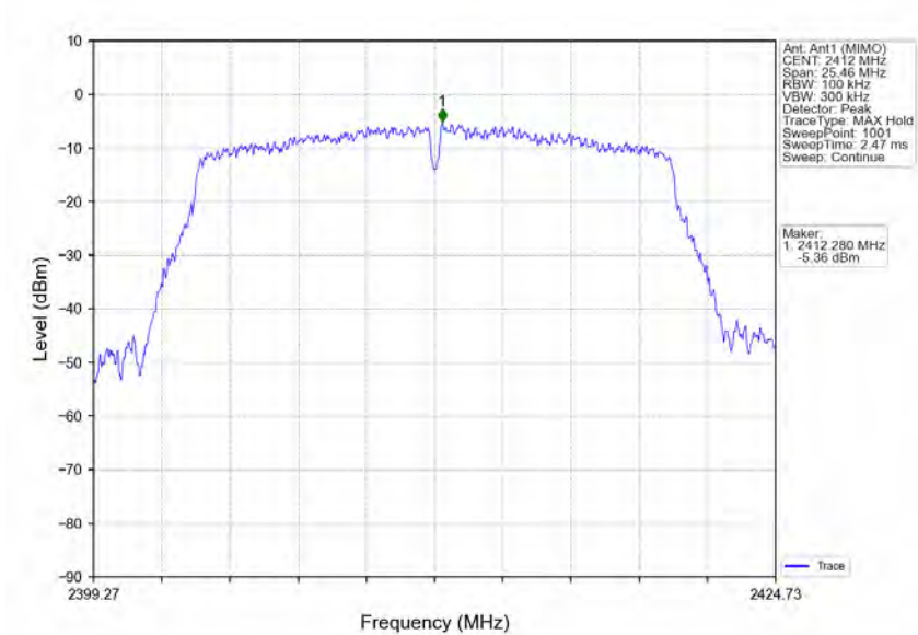
802.11n(HT20) LCH 2412MHz Ant1 (MIMO) NTN
