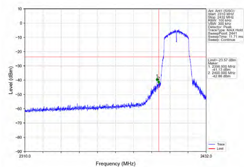
802.11g_LCH_2412MHz_Ant1 (SISO)_NTNV
