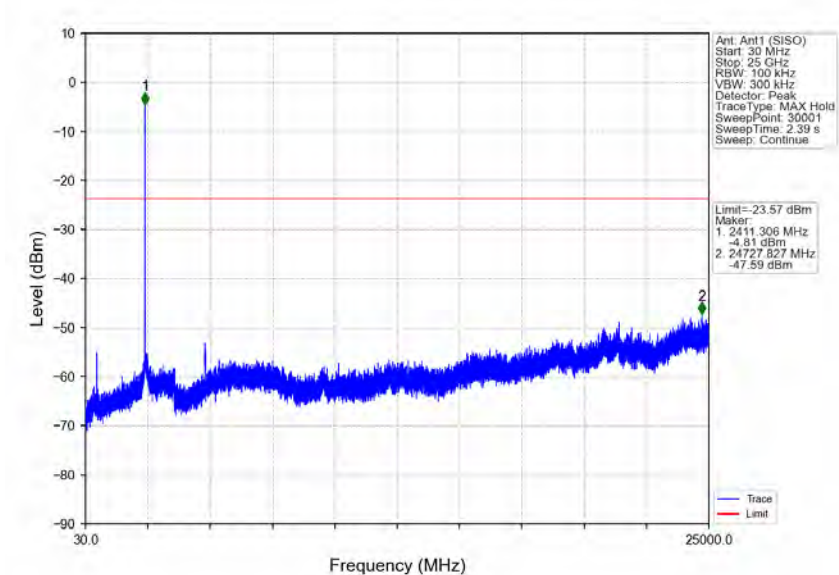
802.11g_LCH_2412MHz_Ant1 (SISO)_NTNV
