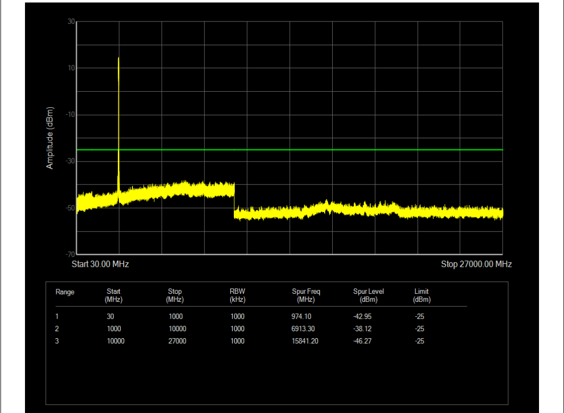
n41 SCS=30kHz DFT_BPSK BW=20MHz Channel=535998 RB=50@0
