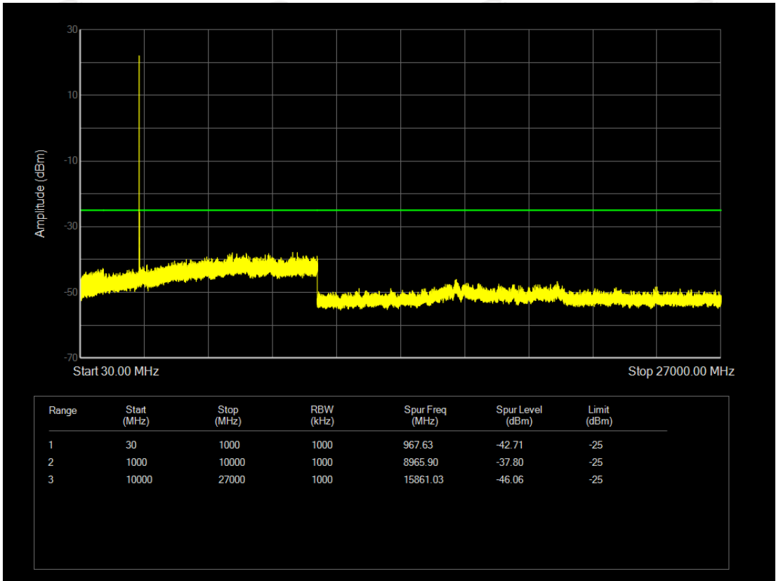
n41 SCS=30kHz DFT_BPSK BW=20MHz Channel=518598 RB=1@0
