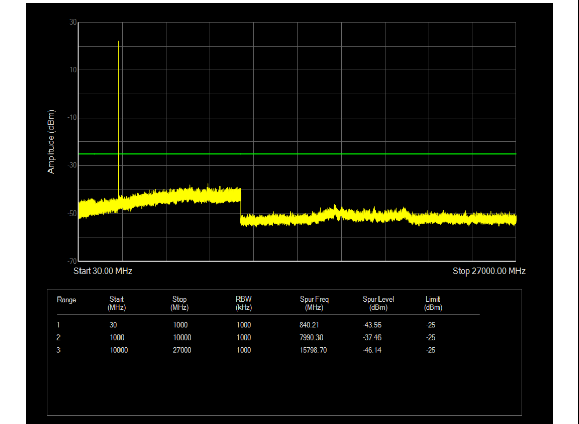
n41 SCS=30kHz DFT_BPSK BW=20MHz Channel=501204 RB=1@0
