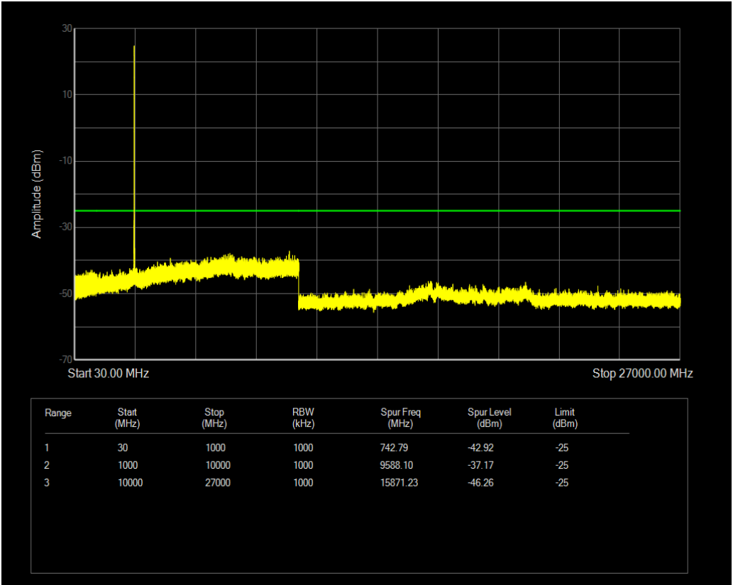
n41 SCS=30kHz DFT_BPSK BW=20MHz Channel=535998 RB=1@0
