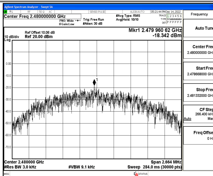
BLE_2M_Ant3_2480
