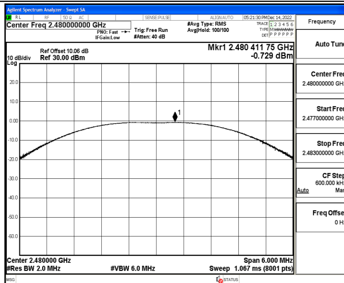
BLE_2M_Ant3_2480
