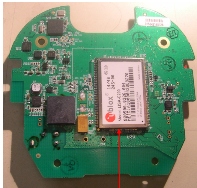
Cell Module
