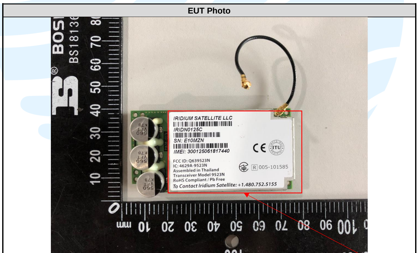
Satellite Module
