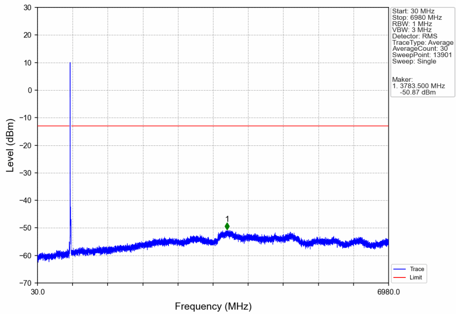
Band71 10MHz 256QAM HCH 693MHz RB 1 0 NTNV
