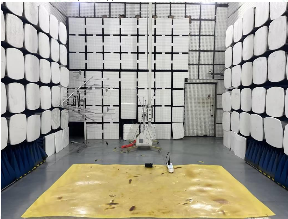
Fig. 1 (30MHz~1GHz)
