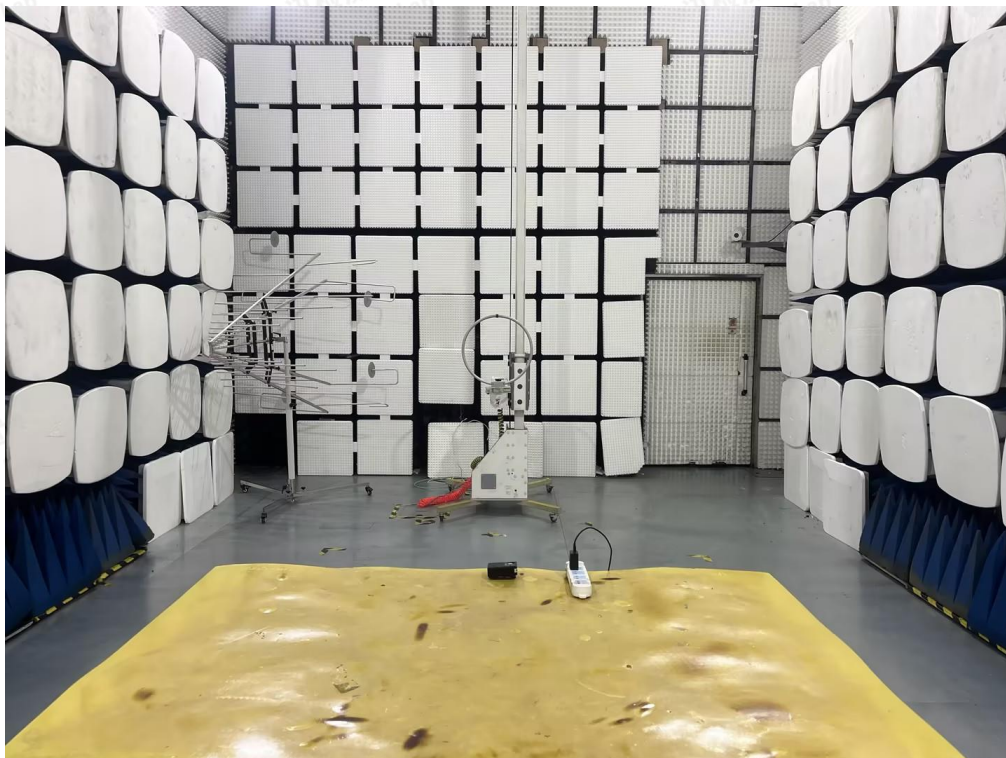
Fig. 3 (Below 30MHz)
