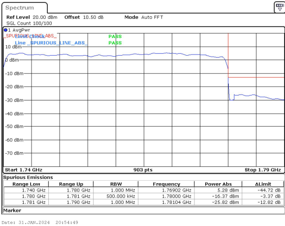
40MHz_15kHz_1760MHz_DFT-s-OFDM QPSK_RB216@0&-16.37 dBm
