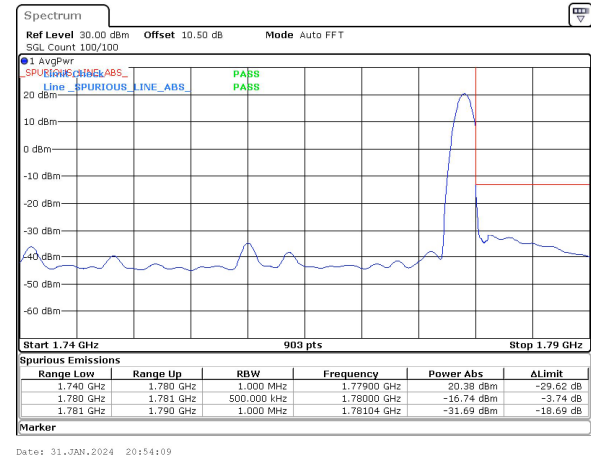
40MHz_15kHz_1760MHz_DFT-s-OFDM QPSK_RB1@215&-16.74 dBm
