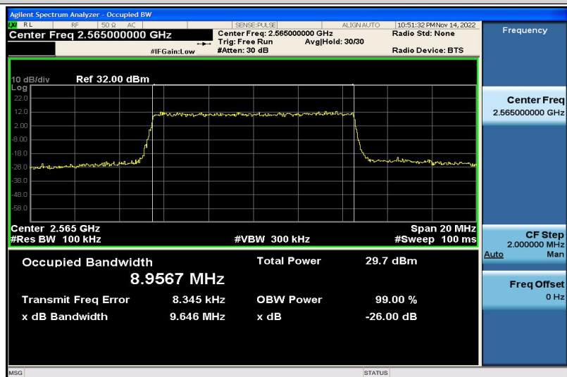
Band7-10MHz-QPSK-21400-50RB#0-8.9567
