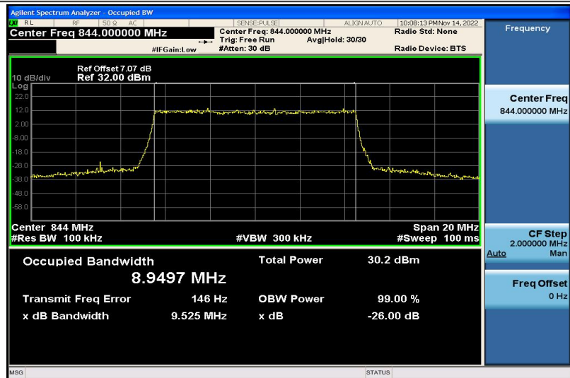
Band5-10MHz-QPSK-20600-50RB#0-8.9497
