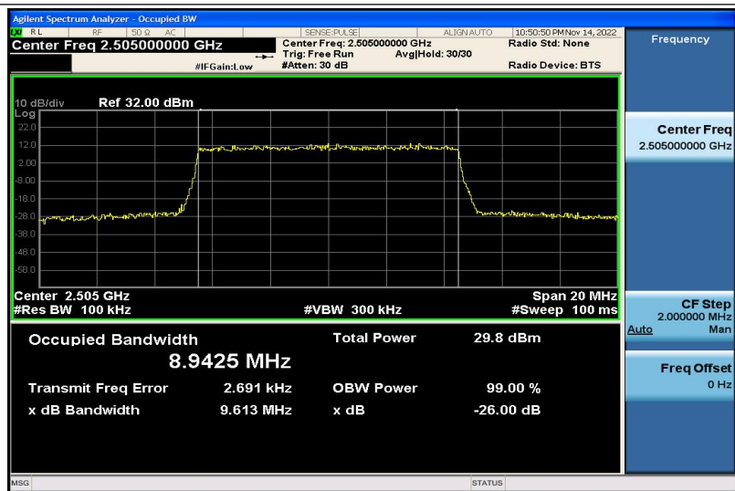
Band7-10MHz-QPSK-20800-50RB#0-8.9425
