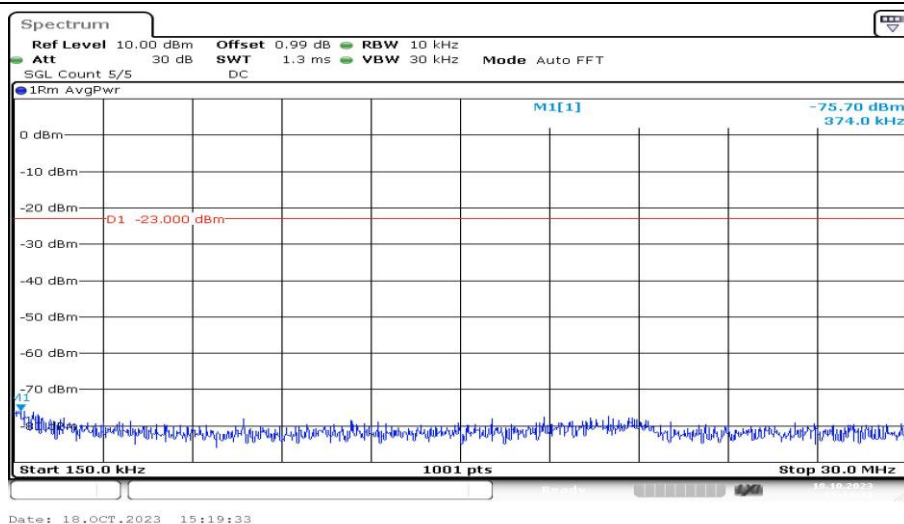
Band12-5MHz-QPSK-23155-1RB#0-Range2:0.15~30MHz-PASS
