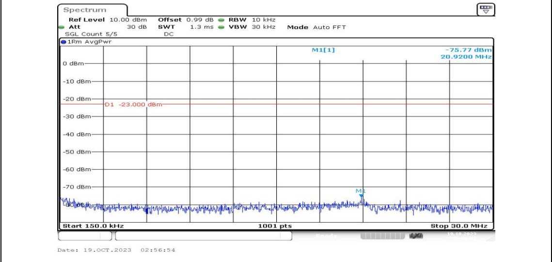
Band12-10MHz-QPSK-23130-1RB#0-Range2:0.15~30MHz-PASS
