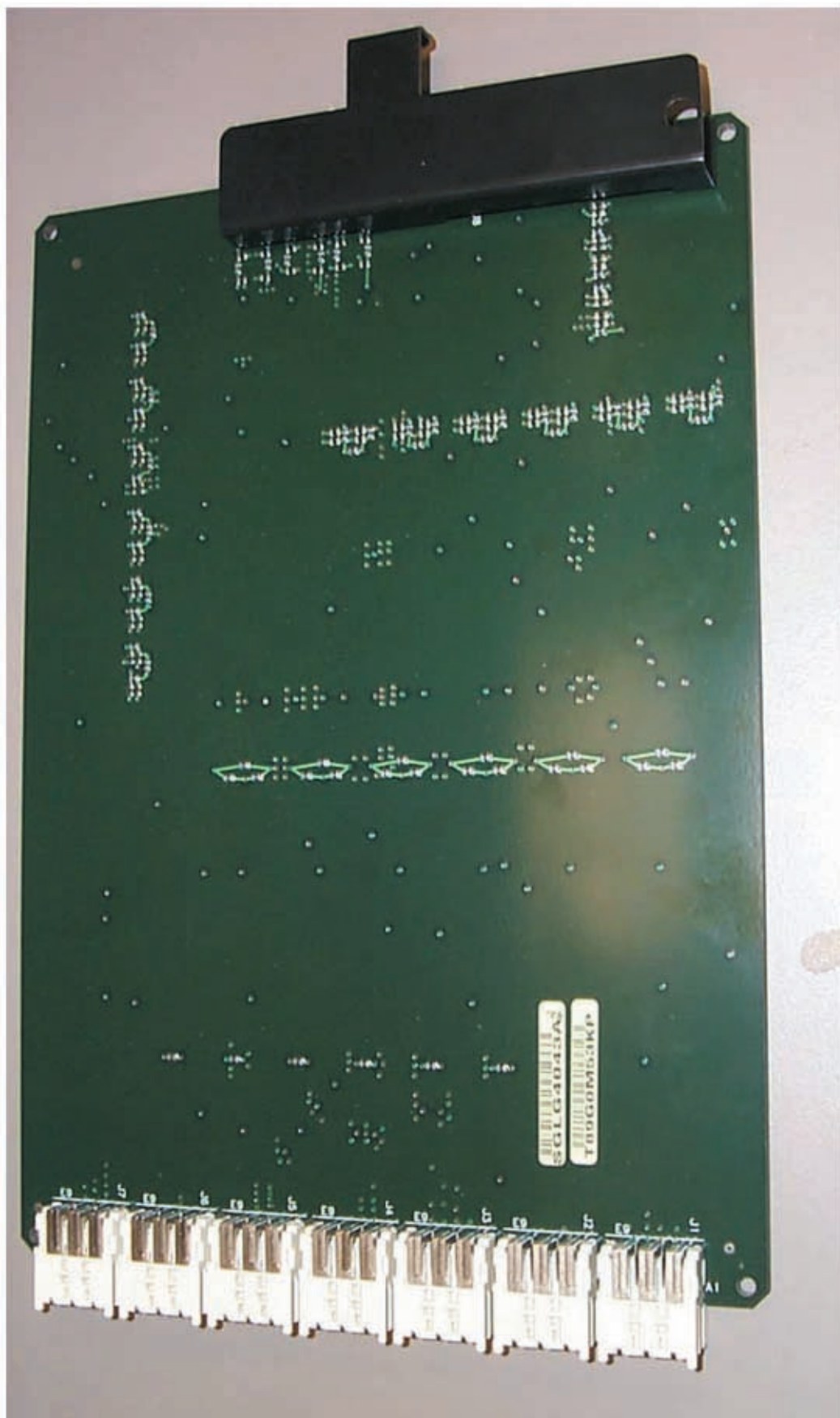
IHET5AP2 4812ETL 800 MHz CIO Front
