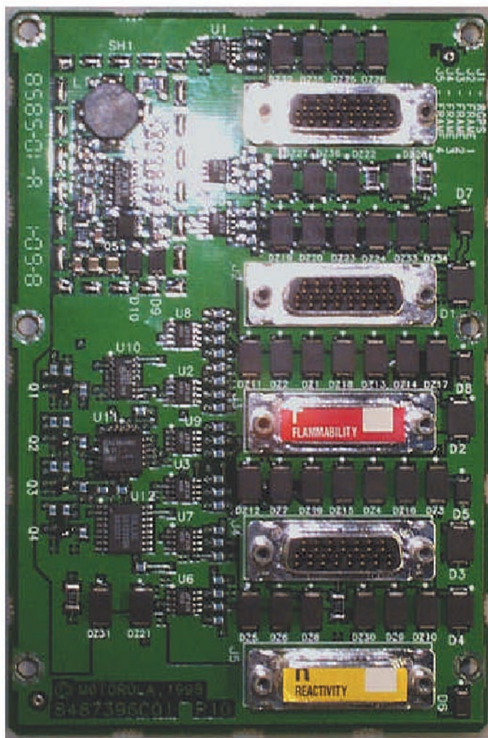
IHET5AP2 4812ETL 800 MHz RGD Front
