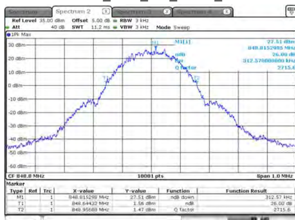
26dB BW_GSM_850_GPRS_848.8
