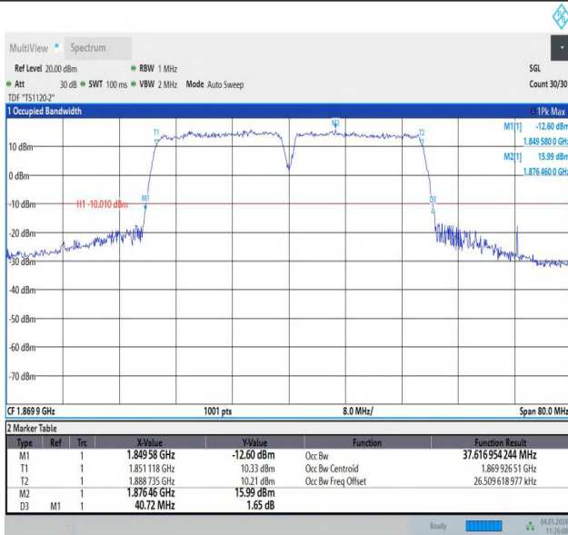
2-2-20MHz-20MHz-QPSK-QPSK-18902-19100-100RB#0-100 RB#0-PASS
