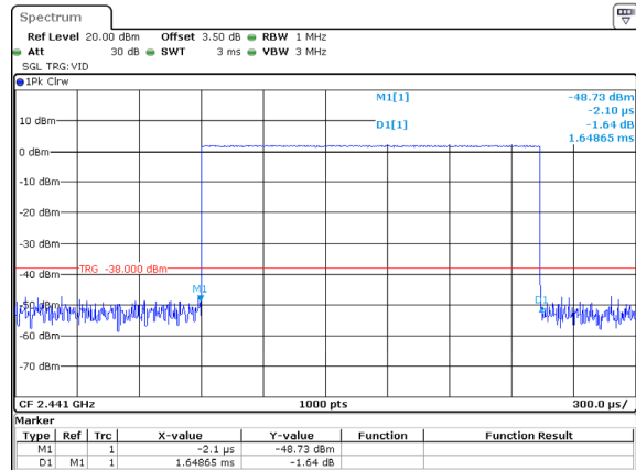
DH3_Hopping 1.649ms
