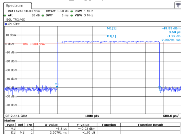
2DH5_Hopping 2.908ms
