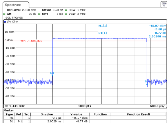
DH5_Hopping 2.903ms
