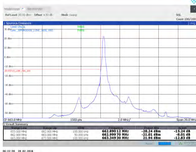
Band71-5MHz-QPSK-133147-25RB#0
