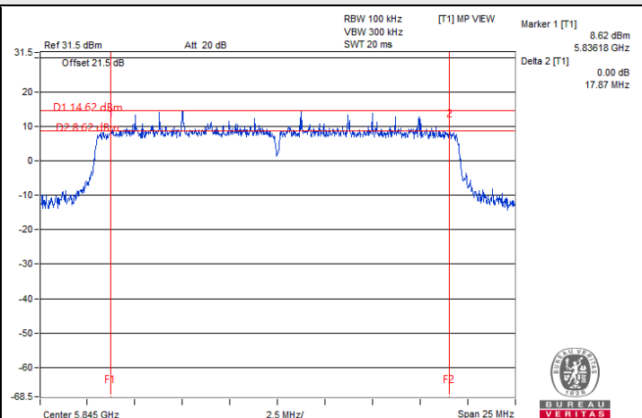
802.11ax (HE20) / Chain 0 : CH 169
