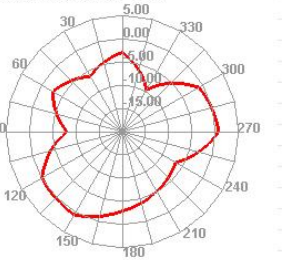
5800.000MHz E2
