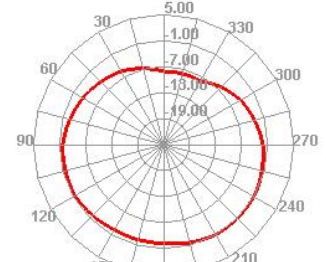
2500.000MHz H
