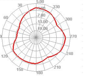
5800.000MHz H
