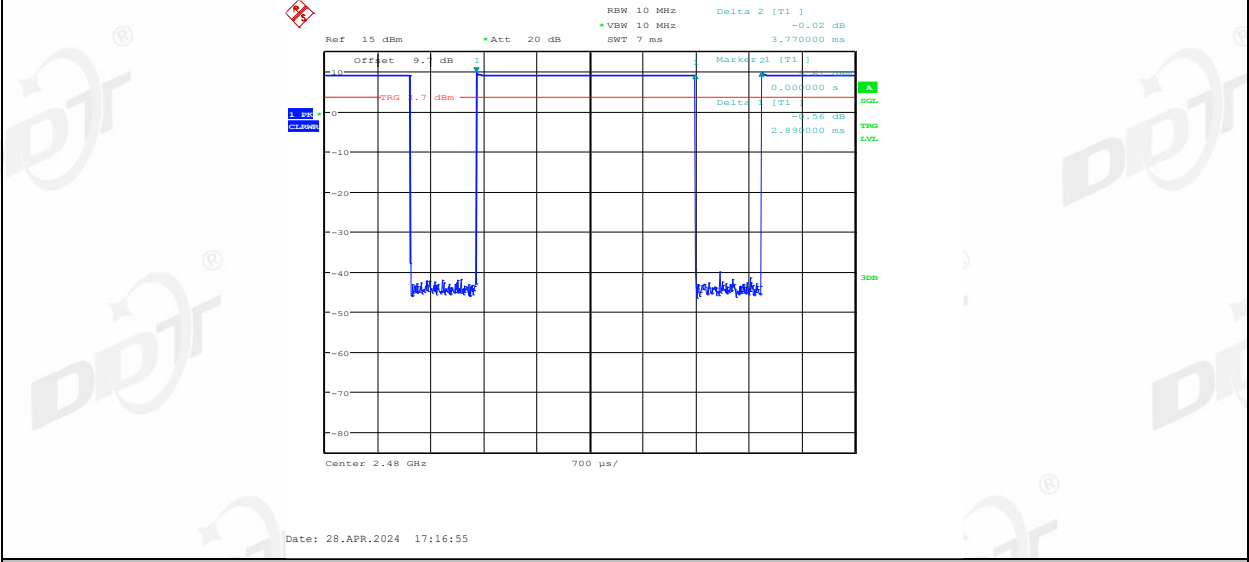
DH5_Left side_2480
