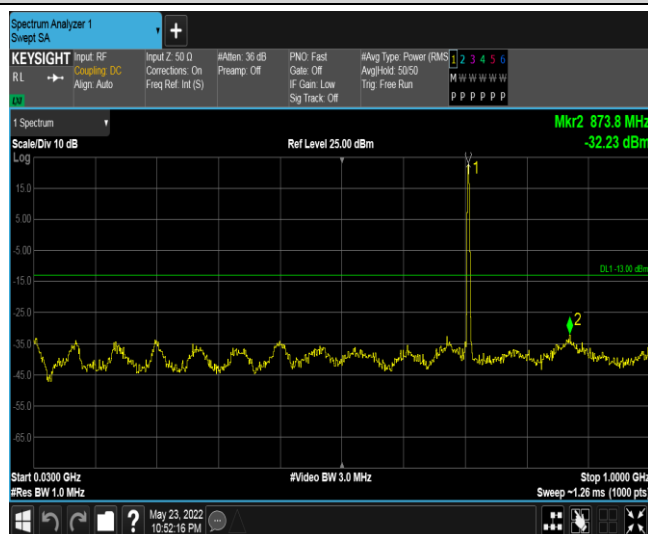
Band12-3MHz-QPSK-23165-1RB#0-Range2:30~1000MHz
