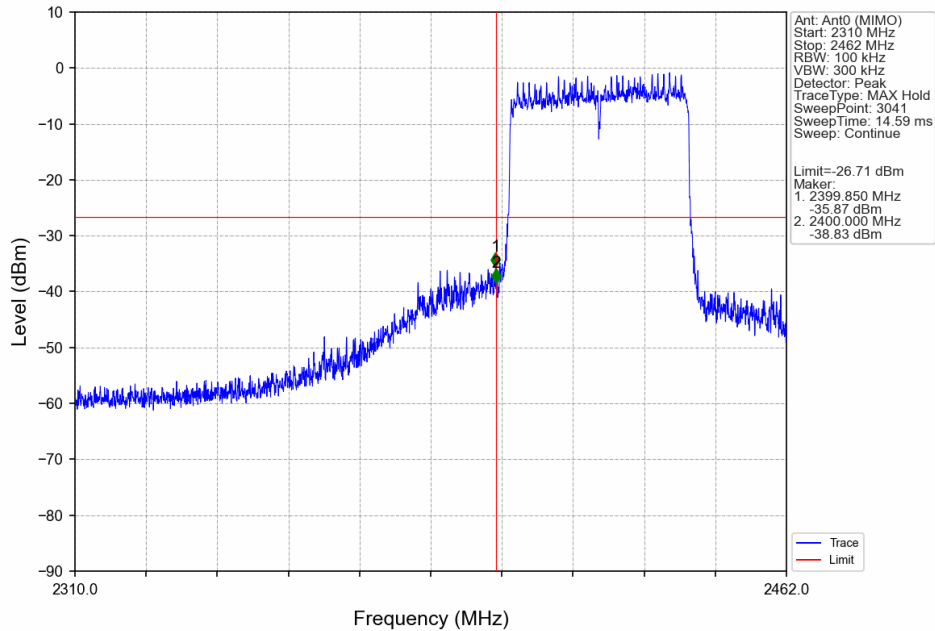
802.11ax(HEW40)_LCH_2422MHz_RU484_Left_Ant0 (MIMO)_NTNV
